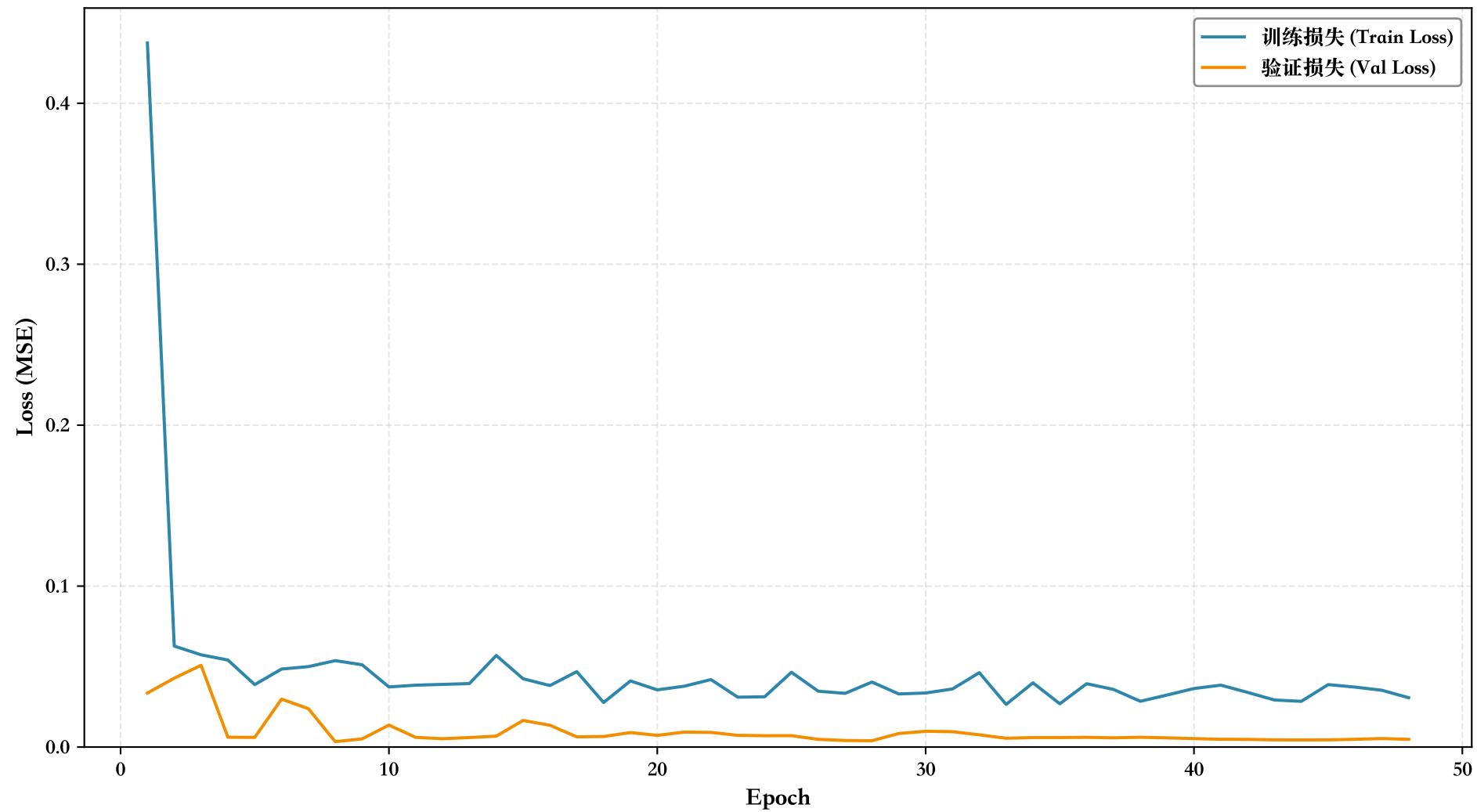
训练/验证损失曲线 - Transformer
