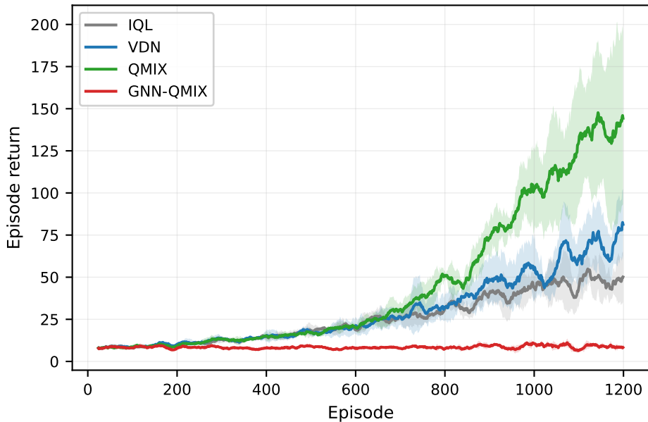
Phase 2 -- CoordGrid (N=8, erdos_renyi)
