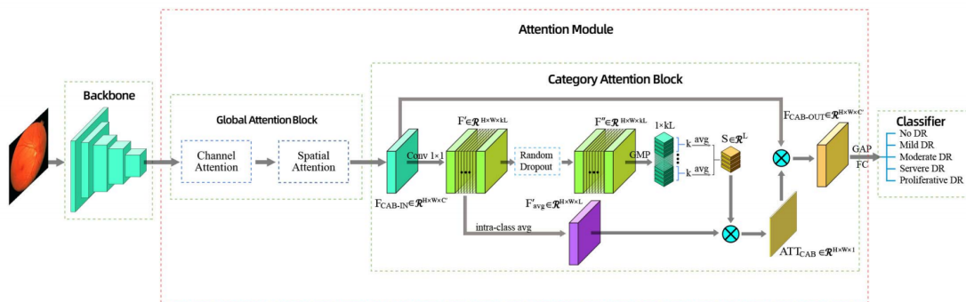
图 4 CABNet 模型结构图 [28]
