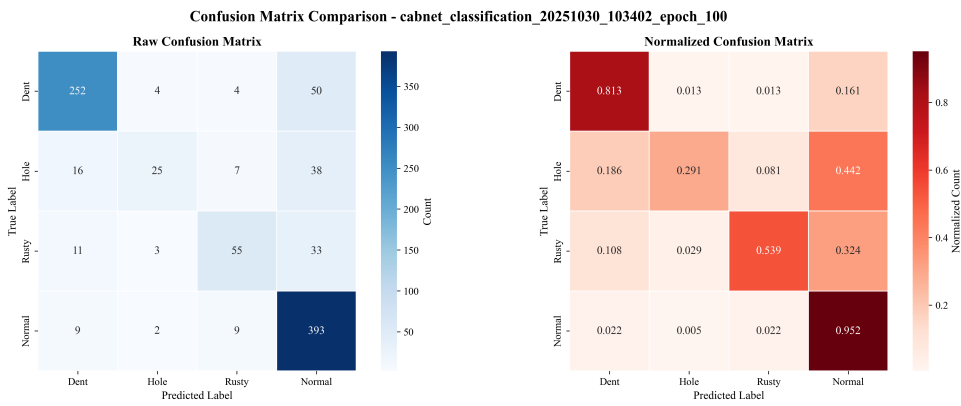
图 15 原始和标准化混淆矩阵对比
