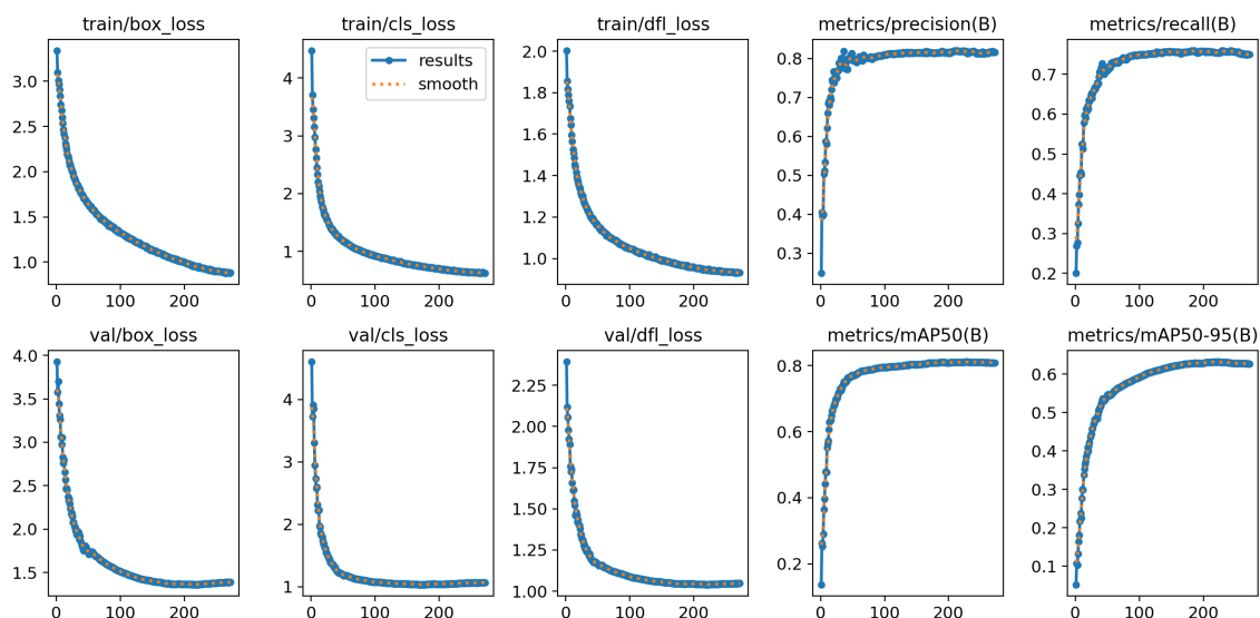
图 10 训练过程中的损失与 mAP 曲线
