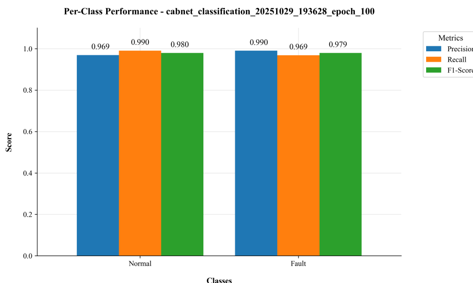
图 8 分类性能指标
