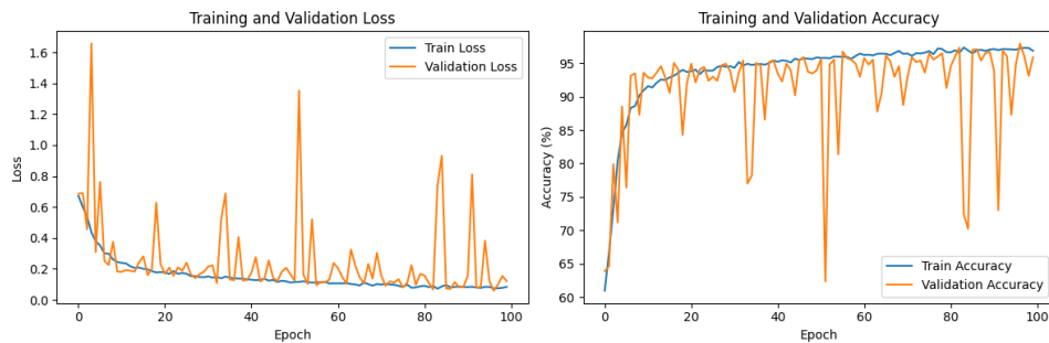
图 6 准确率和损失曲线
