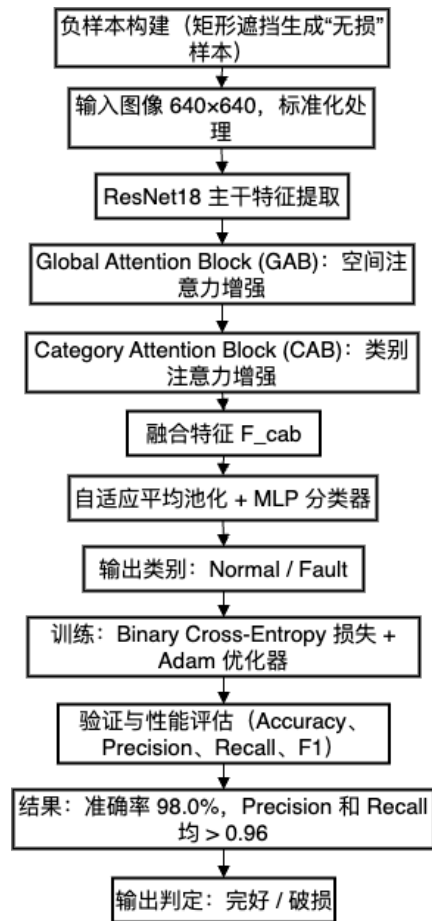
图 5 CABNet 模型训练与评估流程图
