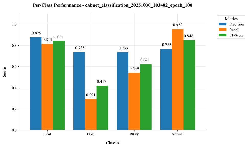
图 16 各类别性能表现对比
