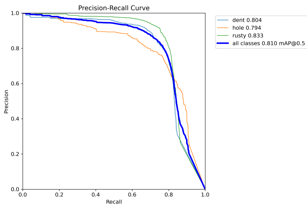
图 11 各类别的 Precision-Recall 曲线
