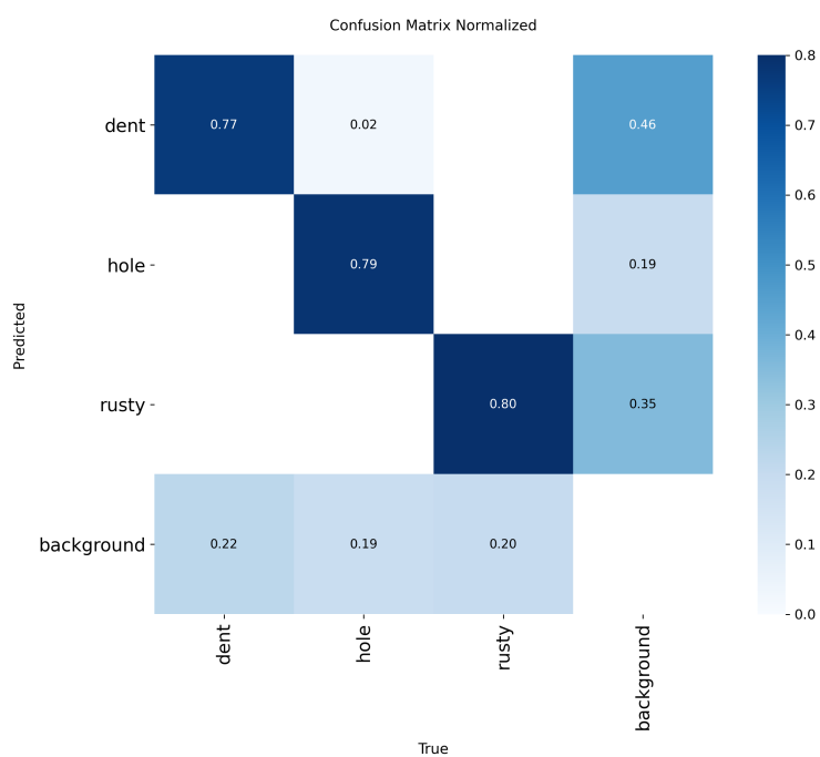
图 12 模型预测结果的混淆矩阵
