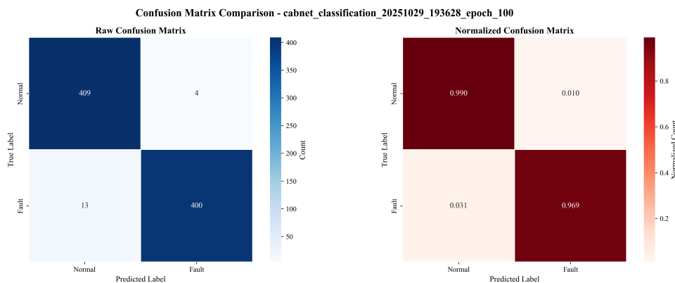
图 7 混淆矩阵
