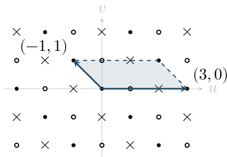
图 9-1: 实心点、空心点、叉号分别表示 u + v 模 3 余 0, 1, 2。箭头标出 H 的基向量, 阴影平行四边形的面积为 3。
