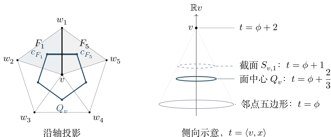
图 3-3: 左图沿原顶点 v 的方向投影。五个邻面 F_i = \text{conv}\{v, w_i, w_{i+1}\} (下标按模 5 计算) 的中心组成蓝色五边形 Q_v ；原边 [v, w_1] 对应加粗的边 [c_{F_5}, c_{F_1}] 。右图区分邻点五边形、面中心五边形与取 \varepsilon = 1 时的顶点截面所在的三个平行平面，椭圆仅示意平面的位置。顶点 v 位于这些平面之外。
