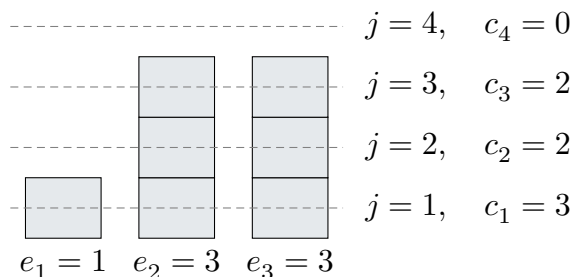
图 9-2: 循环因子指数与层数。柱高是指数 e_i , 第 j 层的柱数是 c_j ; 相邻层数之差数出恰在这一层结束的柱。
