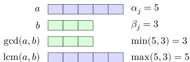
图 11-2: 不可约因子的指数取最小值与最大值。固定一个不可约因子 p_j , 以 \alpha_j = 5 、 \beta_j = 3 为例, 每格表示一个 p_j 因子。
