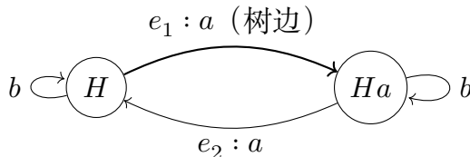
图 8-2: 指数二子群的 Schreier 图。 e_1, e_2 是两条不同的几何边, 指定的正向标签均为 a ; 粗线 e_1 为所选树边。只画正向边, 每条边还有未画出的反向, 其标签为正向标签的逆。
