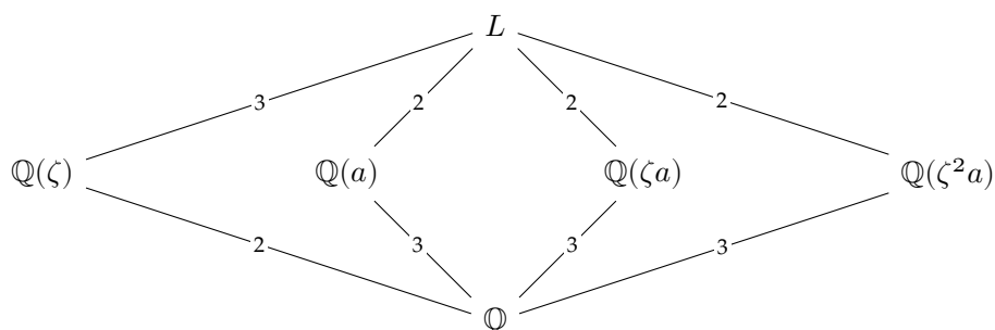
图 19-1: X^3 - 2 分裂域的中问域格。边上的数字为较高的域在较低的域上的次数。
