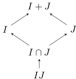
图 10-1: 理想运算的包含关系。 I, J 为同一环的双边理想, 箭头表示包含。
