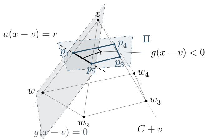
图 3-2: 四棱锥的顶点截面及支持面的提升。蓝色截面位于 \Pi , 灰色平面经过锥顶 v 与截面边 [p_1, p_2] , 其方程为 g(x-v)=0 。截面内的黑色虚线为支持直线 a(x-v)=r , 箭头指向 g(x-v) < 0 的内侧; 延长邻边所得的锥 C+v 全在相应闭半空间内。原面 F_{12} = \text{conv}\{v, w_1, w_2\} 是灰色平面与原多面体的交。
