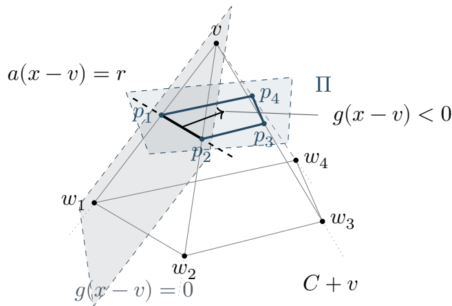
图 3-2: 四棱锥的顶点截面及支持面的提升。蓝色截面位于 \Pi ，灰色平面经过锥顶 v 与截面边 [p_1, p_2] ，其方程为 g(x - v) = 0 。截面内的黑色虚线为支持直线 a(x - v) = r ，箭头指向 g(x - v) < 0 的内侧；延长邻边所得的锥 C + v 全在相应闭半空间内。原面 F_{12} = \text{conv}\{v, w_1, w_2\} 是灰色平面与原多面体的交。
