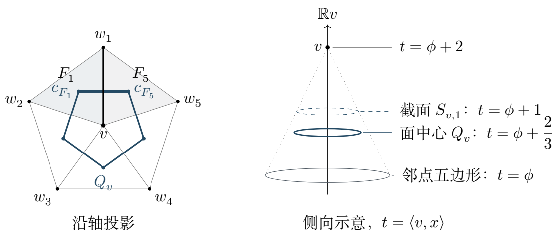
图 3-3: 左图沿原顶点 v 的方向投影。五个邻面 F_i = \text{conv}\{v, w_i, w_{i+1}\} (下标按模 5 计算) 的中心组成蓝色五边形 Q_v ; 原边 [v, w_1] 对应加粗的边 [c_{F_5}, c_{F_1}] 。右图区分邻点五边形、面中心五边形与取 \varepsilon = 1 时的顶点截面所在的三个平行平面, 椭圆仅示意平面的位置。顶点 v 位于这些平面之外。
