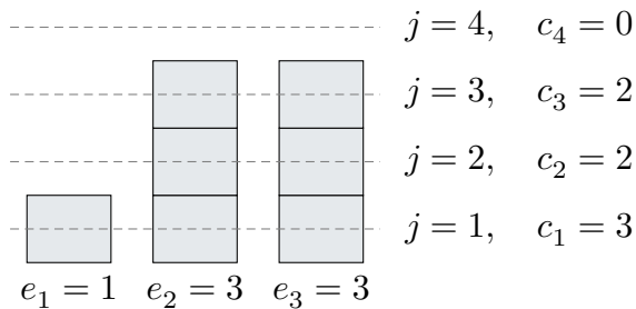
图 9-2: 循环因子指数与层数。柱高是指数 e_i , 第 j 层的柱数是 c_j ; 相邻层数之差数出恰在这一层结束的柱。
