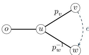
图 8-1: 实线是生成树中的边, 虚线是非树边 e: v \rightarrow w 。树路径 p_v: o \rightarrow u \rightarrow v 与反向树路径 p_w^{-1}: w \rightarrow u \rightarrow o 共用 o, u 之间的边; 对应的自由元素是闭路径类 [p_v e p_w^{-1}] 。
