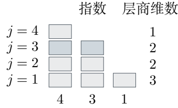
图 4-1: 主分量层商与初等因子。列高为 4, 3, 1, 着色的第三层有两个格子, 第四层有一个格子, 二者之差说明指数恰为 3 的循环分量有一个。
