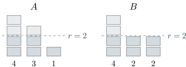
图 1-1: Jordan 块的层数与幂核维数。每列高度是块大小，着色的两层分别有 5 与 6 个格子，对应 \dim \ker A^2 与 \dim \ker B^2 。
