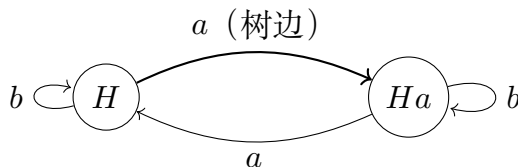
图 8.1: 指数二子群的 Schreier 图。只画指定的正向边, 粗线表示所选树边。每条边还有未画出的反向, 其标签为正向标签的逆。
