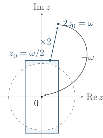
图 11-1: 格点引理中的基本矩形与单位圆 (虚线)。阴影为矩形内满足 |z_0| \geq 1 的上下两片区域; 箭头分别表示倍乘与减去格点, 图中展示的是零余数实例。
