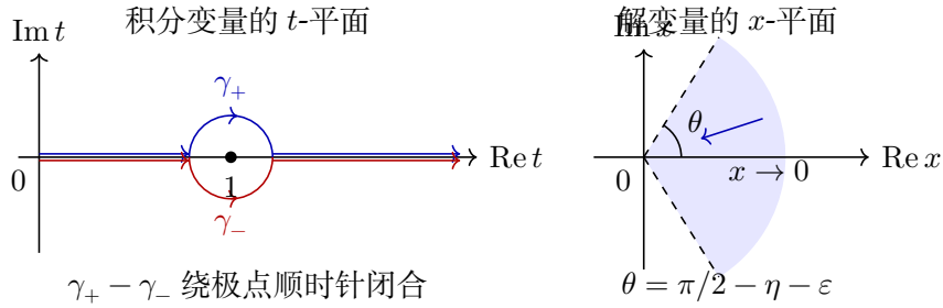
图 D-1: Stokes 算例中的两个复平面。左图的路径绕开积分极点；右图的扇形使沿这些路径的 e^{-t/x} 衰减，且 e^{-1/x} 在 x \rightarrow 0 时指数衰减。
