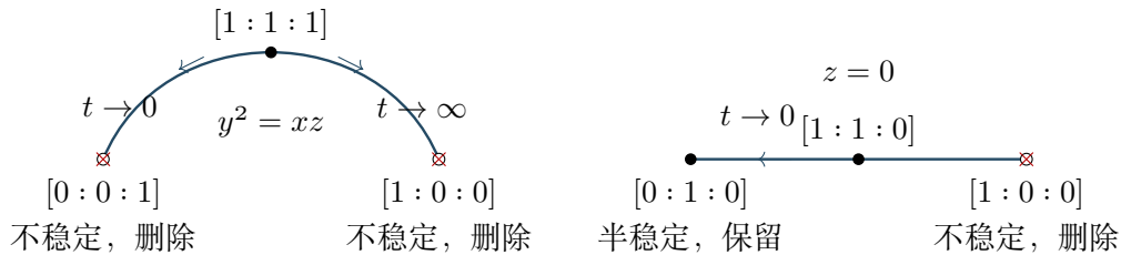
图 22-1: 两个射影轨道闭包及其边界点的示意。左侧轨道的两个边界点都不在半稳定集中, 右侧轨道却留下一个半稳定边界点。空心叉号表示删除的点, 实心点表示保留的点; 曲线形状仅用于示意闭包中的包含关系。
