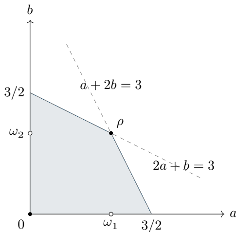
图 18-1: 以基本权系数 (a, b) 为坐标, 阴影表示支配室与 \rho - \sum_i \mathbb{R}_{\geq 0} \alpha_i 的交。其中四个整数点只有两个黑点满足根格陪集条件; 两个空心点不满足。
