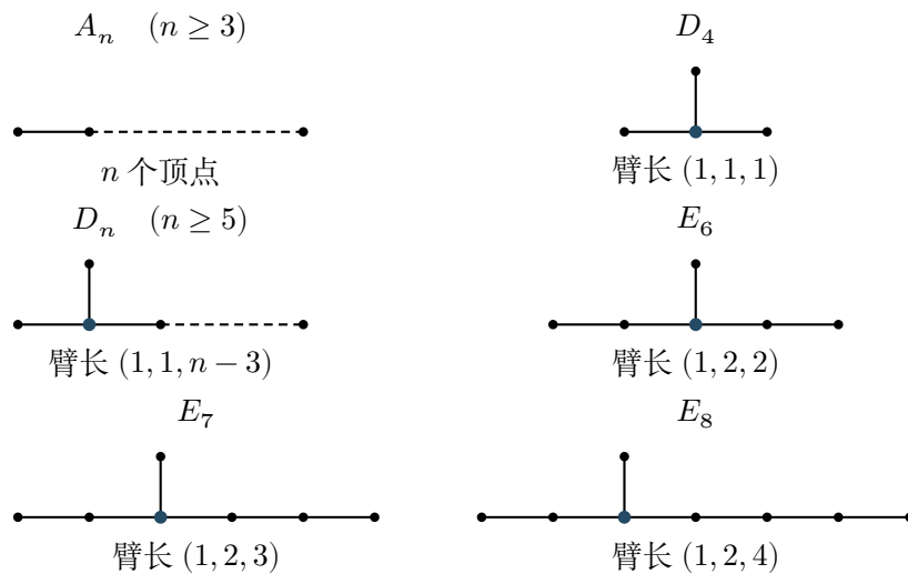
图 10-1: ADE 图及臂长。蓝色顶点为三叉点，臂长计中心之外的顶点数。虚线表示链段，其中可以没有额外顶点： A_3 与 D_5 的虚线各是一条边。 A_1 是单顶点， A_2 是单边； D_4 的三条臂均长 1。
