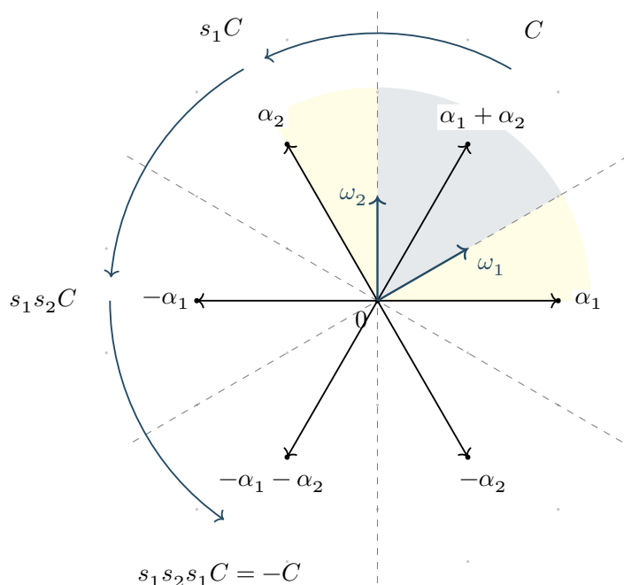
图 17-1: A_2 的六根、三条墙及室链。淡黄色扇形是正简单根实锥, 蓝色扇形是基本室; 二者的边界不同。灰点表示权格, 黑点表示根格。 \omega_1 位于垂直于 \alpha_2 的墙上, 故被 s_2 固定。外侧箭头给出到相反室的三步最短室链。
