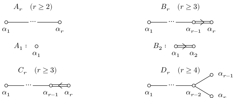
图 17-2: 经典 Dynkin 图。省略号表示可含零个中间顶点的单边链段，根的编号沿链递增。双边箭头指向短根； D_r 的分叉点为 \alpha_{r-2} 。
