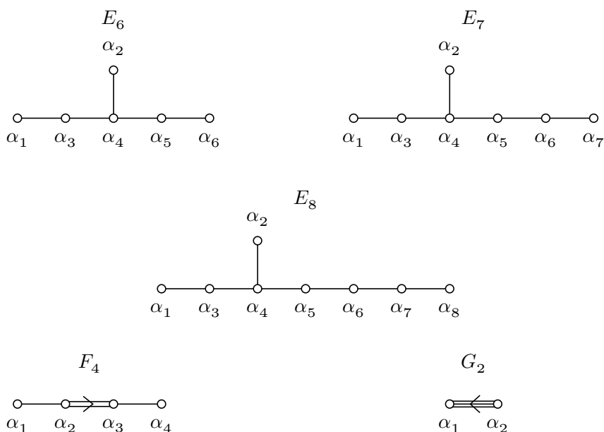
图 17-3: 例外型 Dynkin 图。 E_6, E_7, E_8 的分叉点均为 \alpha_4 ，三个臂长分别为 (1, 2, 2) 、 (1, 2, 3) 、 (1, 2, 4) ；臂长计中心之外的顶点数。 F_4 的末两根短， G_2 的第一根短。
