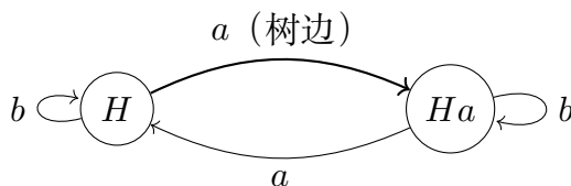
图 8.1: 指数二子群的 Schreier 图。只画指定的正向边, 粗线表示所选树边。每条边还有未画出的反向, 其标签为正向标签的逆。
