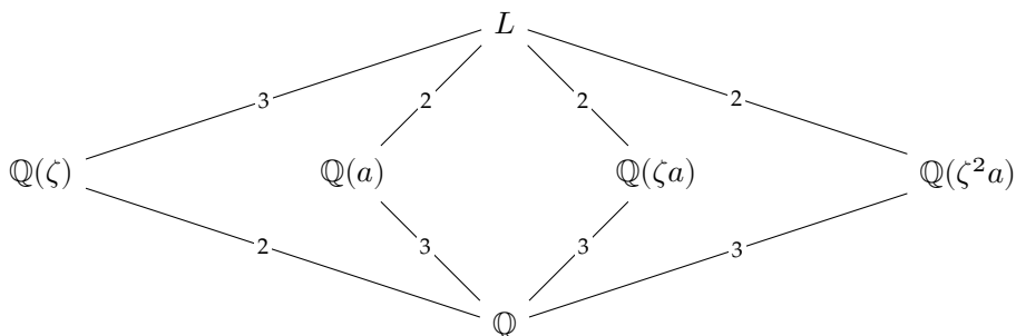
图 19-1: X^3 - 2 分裂域的中间域格。边上的数字为较高的域在较低的域上的次数。
