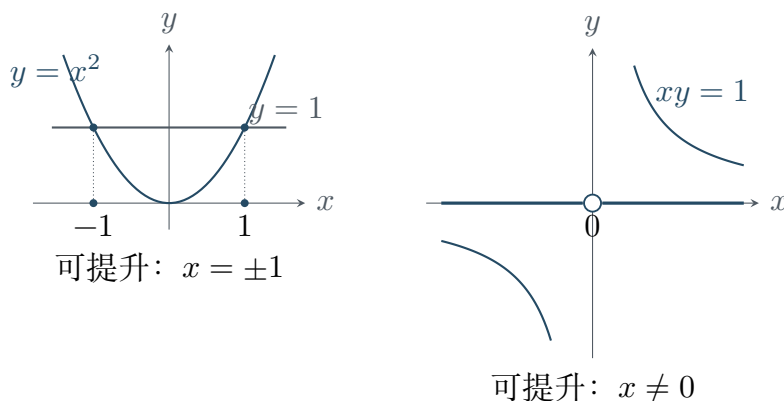
图 12-1: 两个实数点例子。左：消去方程 x^2 - 1 = 0 的两个实根都能提升到交点；右：消去理想为零，故消去方程不排除 x = 0 ，但 xy = 1 的实数解只有非零的第一坐标。满足消去方程只是原方程组有解的必要条件。
