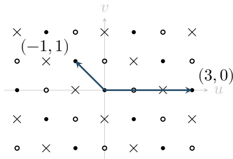
图 9-1: 实心点、空心点、叉号分别表示 u+v 模 3 余 0, 1, 2。箭头标出 H 的基向量。
