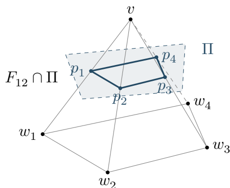
图 3-2: 以四棱锥为例说明顶点截面。原邻边 [v, w_i] 与切割平面 \Pi 相交于截面顶点 p_i ; 经过 v 的面 F_{12} = \text{conv}\{v, w_1, w_2\} 在截面中给出边 [p_1, p_2] 。正文引理适用于任意有限条邻边。
