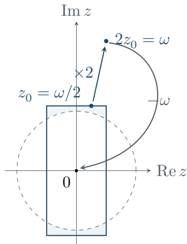
图 11-1: 格点引理中的基本矩形与单位圆 (虚线)。阴影为矩形内满足 |z_0| \geq 1 的上下两片区域; 箭头分别表示倍乘与减去格点, 图中展示的是零余数实例。
