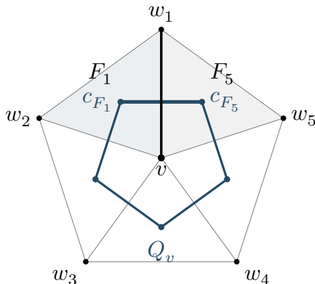
图 3-3: 沿原顶点 v 的方向观察的局部投影。五个邻面 F_i = \text{conv}\{v, w_i, w_{i+1}\} (下标按模 5 计算) 的中心组成蓝色五边形 Q_v 。原边 [v, w_1] 邻接 F_5, F_1 , 对应加粗的边 [c_{F_5}, c_{F_1}] 。
