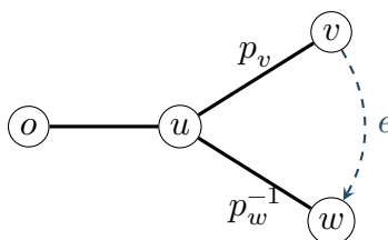
图 8-1: 实线是生成树中的边，虚线是非树边 e: v \rightarrow w 。树路径 p_v: o \rightarrow u \rightarrow v 与反向树路径 p_w^{-1}: w \rightarrow u \rightarrow o 共用 o, u 之间的边；对应的自由基元素是闭路径类 [p_v e p_w^{-1}] 。
