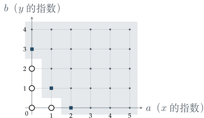
图 F-1: J = (x^2, xy, y^3) 的指数阶梯, 图中只画出有限范围。方块表示生成元的指数 (2,0), (1,1), (0,3) ; 着色区域中的整数点对应 J 的单项式, 空心圆对应 1, x, y, y^2 。图中是单项式的指数点, 并非由 J 给出的方程组的解点。
