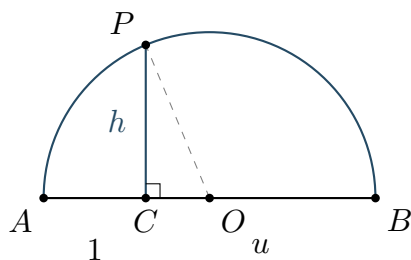
图 21-1: 半圆开平方作图。 AC = 1 、 CB = u > 0 , O 为 AB 的中点, 过 C 的垂线与上半圆交于 P 。高度 CP = h 满足 h^2 = u 。图形比例仅作示意。
