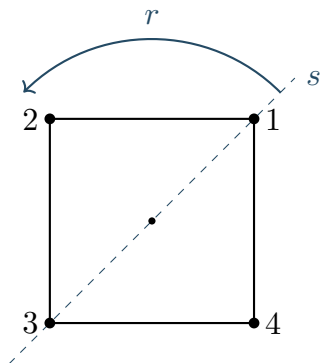
图 3-1: 正方形的旋转与反射。逆时针四分之一周旋转为 r = (1234) ，沿虚线的反射为 s = (24) 。先反射、再旋转、再反射，得到反向旋转，即 srs = r^{-1} 。
