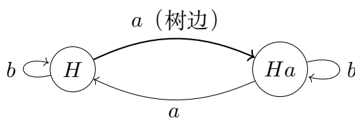
图 8-2: 指数二子群的 Schreier 图。只画指定的正向边, 粗线表示所选树边。每条边还有未画出的反向, 其标签为正向标签的逆。
