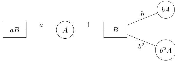
图 C-1: C_2 * C_3 陪集树中单位边附近的部分。圆形表示 A 型顶点，方形表示 B 型顶点；顶点标签是左陪集，边标签是群元素。边界处的顶点仍继续向外连接。
