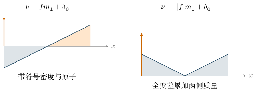
图 6.1: 符号测度的正负质量与全变差. 这里 f = (2x - 1) \cdot \mathbf{1}_{[0,1]} . 折线表示连续部分的密度, 箭头表示单位原子. 箭头高度仅用于辨认原子, 不与密度纵坐标作面积比较.
