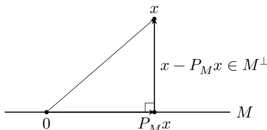
图 8.2: Hilbert 投影。向量 x 唯一分解为 M 内的最佳近似 P_M x 与正交误差 x - P_M x 。
