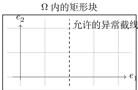
图 21.1: ACL 坐标截线。实线示意良好截线, 虚线只表示某个允许排除的截线; 真正的例外族由横向零测集参数化。
