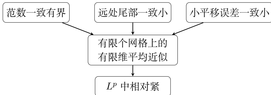
图 25.1: 平移紧性机制。三个条件分别控制平均值大小、需要保留的空间范围和网格尺度。
