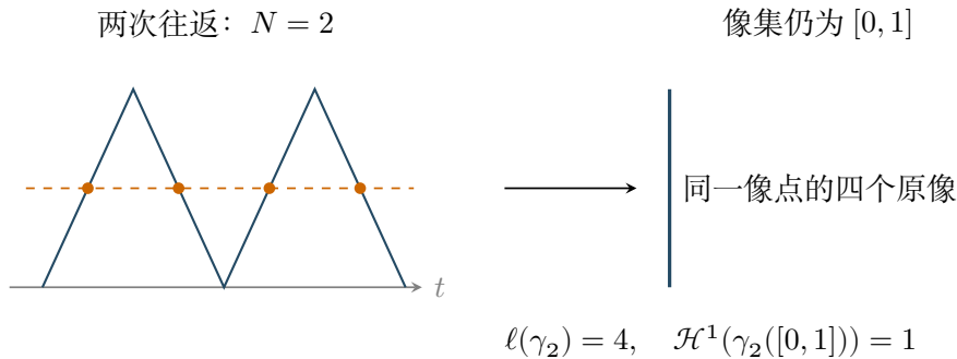
图 17.2: 参数重复经过与重数计数。取既有往返曲线习题中的 N = 2 。几乎每个像点经过四次, 故长度等于像上重数的积分, 而非像集长度。
