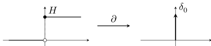
图 20.2: 跳跃的分布导数。Heaviside 函数的变化集中在原点，故 \partial T_H = \delta_0 。
