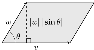
图 17.1: Gram 面积。由 v, w 张成的平行四边形面积为 \sqrt{\det G} = |v| |w| |\sin \theta| 。
