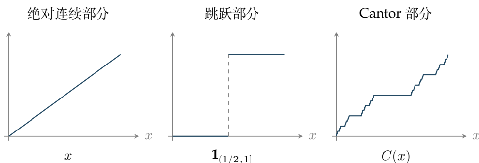
图 28.1: 体积、跳跃与 Cantor 变化。图示三个函数; 在 (0, 1) 上把它们相加, 导数分别产生 Lebesgue 测度、一个原子和 Cantor 测度。右图为有限分辨率示意, 不将 Cantor 测度画成普通密度。
