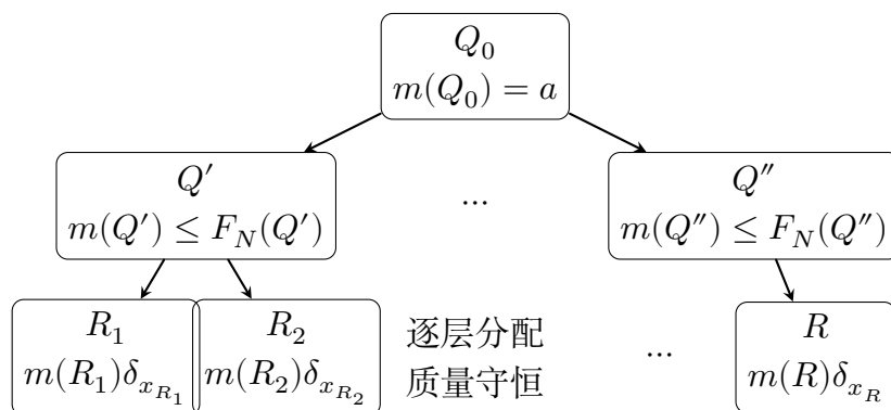
图 15.3: 二进质量分配。根质量 a 逐层向子立方体分配; 每个结点受容量 F_N 控制, 末层质量则变成位于 K 上的原子。图中只画出部分分支。
