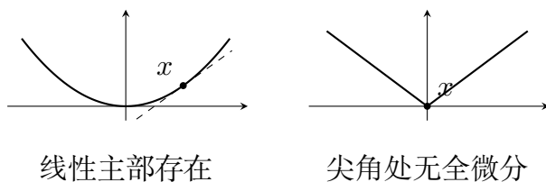
图 16.1: 可微点与尖角。左图的虚线表示一阶线性近似；右图说明 Lipschitz 条件仍允许出现不可微点。
