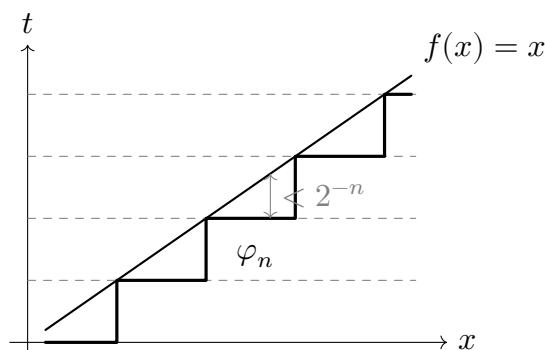
图 4.1: 二进简单逼近。阶梯函数在每个二进小区间取左端点值，始终不超过 f ，并随网格加密从下方逼近。
