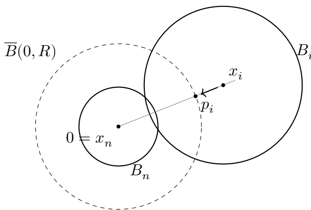
图 13.2: 径向压缩。与末球 B_n 相交的旧球中心 x_i 若位于 \overline{B}(0, R) 外, 就沿射线压到 p_i ; 证明的核心是这些压缩点仍有统一的分离距离。示意图不按比例。
