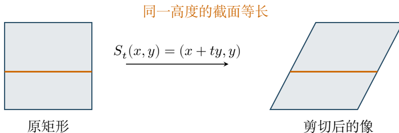
图 3.1: 剪切为什么保持体积。剪切保留水平截面的长度；由非负截面积分得到面积不变。图示为正剪切参数的一个情形。
