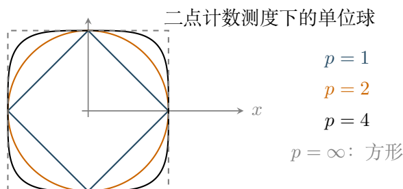
图 10.1: 二点空间上的 L^p 单位球。二点空间上的 L^p 范数就是 \ell^p 范数。单位球分别呈菱形、圆、圆角方形和方形; 有限维图不说明一般 L^p 的弱紧性。
