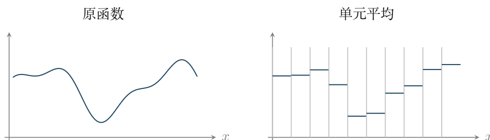
图 25.2: 网格平均与有限维逼近。有限区间上的网格平均示意。一般 L^p 论证先控制空间尾部，再以平移估计控制网格平均误差；最后保留的网格数有限。
