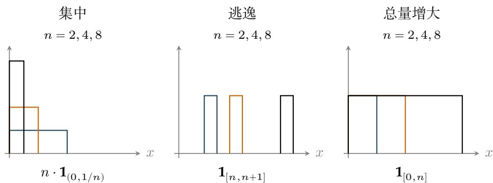
图 5.1: 集中、逃逸与幅值尾部。集中族的积分恒为一且不一致可积；后两族按本书幅值尾部定义均一致可积，但分别存在空间逃逸和积分总量无界。各面板坐标尺度不同。
