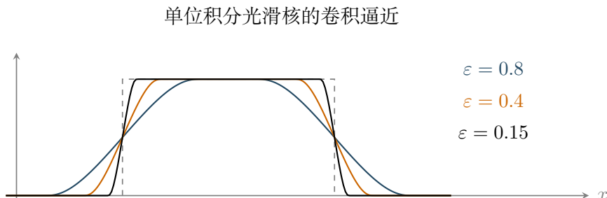
图 20.1: 卷积如何移动、平均与光滑化。虚线为区间示性函数；实线为它与尺度化光滑核的卷积。核取 C \exp(-1/(1-x^2)) 于 |x| < 1 ，区间外为零，其中常数使积分为一。
