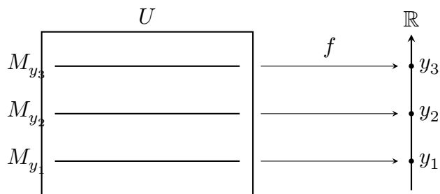
图 18.1: 水平集切片。投影 f(z, w) = w 把每张平行水平集 M_y 压到目标空间中的一点 y 。
