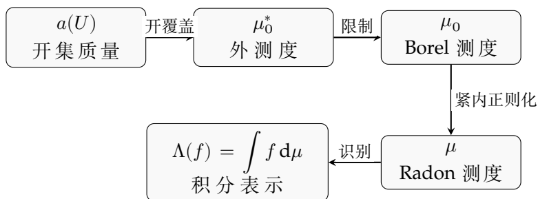
图 11.1: 表示测度的构造。从开集候选质量到积分表示, 中间的 \mu_0 与 \mu 分别承担外逼近和紧内正则化。
