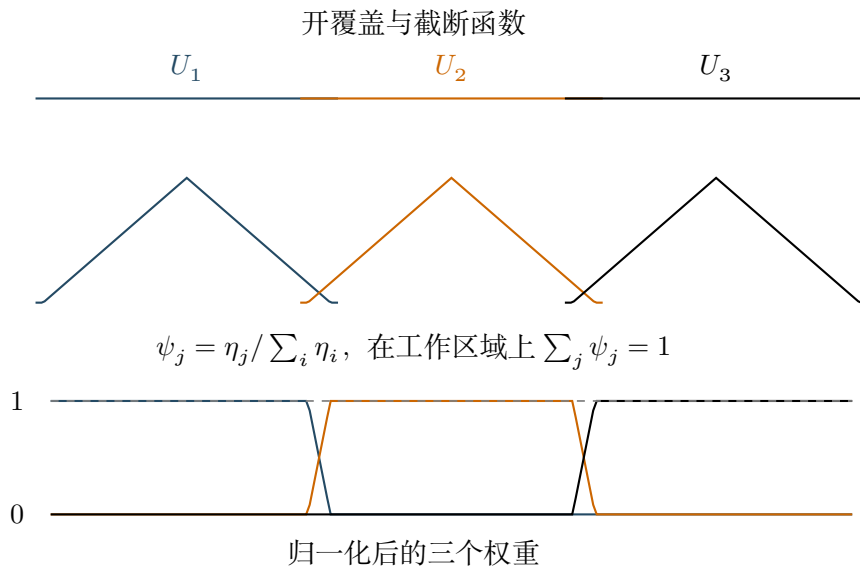
图 22.2: 局部覆盖与单位分解拼接。折线仅示意非负截断的支撑与重叠, 实际选取光滑截断。分母在工作区域上为正, 归一化后权重和为一; 可数情形还需局部有限性。
