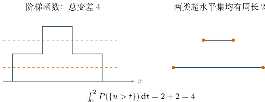
图 27.1: BV 的层集与周长积分。一维紧支集阶梯模型在每个非临界层值都有两个边界点。变差把跳跃高度计入, 而每层周长只计边界。
