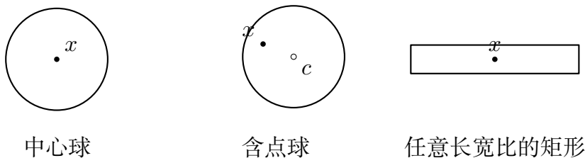
图 13.4: 三类微分基。前两类保持球形, 但观察点与球心的关系不同; 第三类若不限制长宽比, 偏心率可以任意增大。
