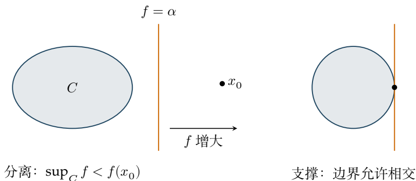
图 8.1: 凸分离与支撑泛函。左图示意实泛函的严格分离；右图示意支撑超平面。二维欧氏图只解释几何位置，不要求一般分离泛函来自正交投影。
