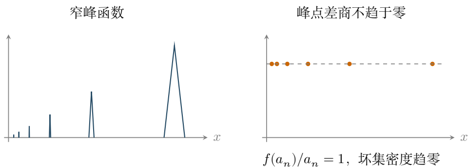
图 16.2: 稀疏尖峰与近似微分。使用本章习题的参数 a_n = 2^{-n} 、 b_n = a_n^2/8 。左图画出了前六个三角峰；全部峰的支撑在原点密度为零，但峰点差商恒为一。
