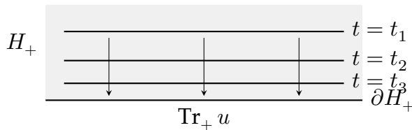
图 23.1: 半空间迹。内部切片 u(\cdot, t) 随 t \downarrow 0 在 L^p 中趋向边界数据 \text{Tr}_+ u 。
