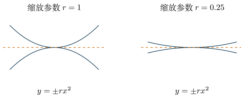
图 19.2: 相切曲线的同一切线与重数二。两条曲线在原点有同一近似切线, 但每支贡献一份长度, 密度为二, 缩放极限带重数二。这不反驳几乎处处的单位密度结论。
