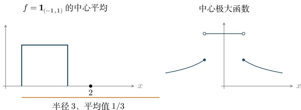
图 13.3: 移动平均与极大函数的超水平集。对中心极大算子, Mf 在开区间内为一, 在 |x| \geq 1 时为 1/(1+|x|) 。端点值是二分之一; 非中心版本不能套用这条曲线。
