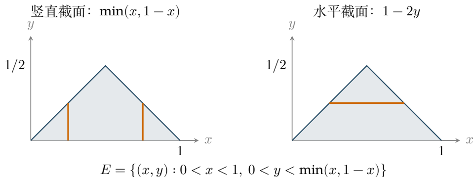
图 7.1: 同一积分域的两片切片。同一三角域按两种方向切片, 截面长度的积分均为四分之一。边界为零测, 不影响本题面积。
