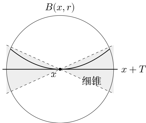
图 19.1: 近似切平面。灰色区域表示围绕仿射平面 x + T 的细锥；锥外质量在缩放后可以忽略。
