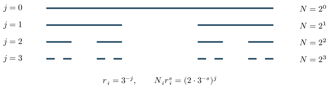
图 15.1: 覆盖尺度与 Hausdorff 维数。自然覆盖的代价在 s = \log 2 / \log 3 两侧表现不同。图只展示这些覆盖的上界机制；维数的反向估计仍需质量分布等论证。
