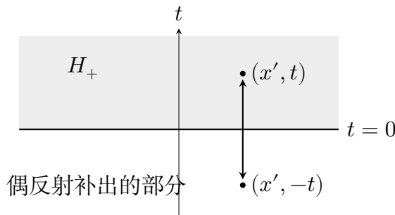
图 22.1: 半空间偶反射。定义 E_+u(x', -t) = u(x', t) , 函数值跨边界接合, 而法向导数改变符号。
