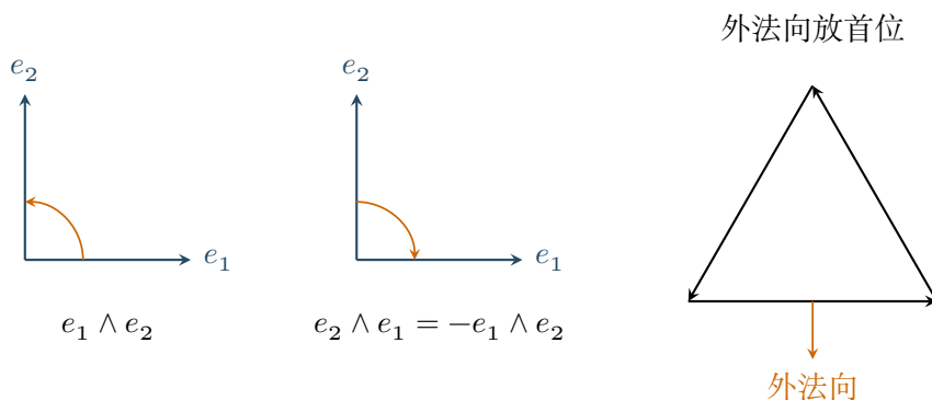
图 B.1: 定向、换基与边界方向。交换有向基的次序改变外积符号; 右图采用平面的标准定向, 边界逆时针, 外法向在有序基中放首位。
