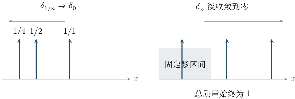
图 12.1: 原子测度的汇聚与质量逃逸。每根箭头都代表单位质量。逃逸族的紧支集测试趋零，但常函数一的积分不变，因此它不弱收敛到零测度。
