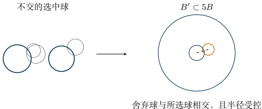
图 13.1: 5r 选球与膨胀覆盖。左图为有限选球示意；右图把一个选中球放大显示，外圆半径是内圆的五倍。覆盖结论仍依赖证明中的选取顺序与半径比较。
