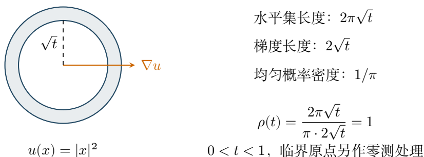
图 18.2: 径向水平集与余面积分母。二维单位圆盘上的均匀分布经 |x|^2 推前后，在 (0, 1) 上密度为一。薄环的面积与层值宽度之间由梯度长度连接。
