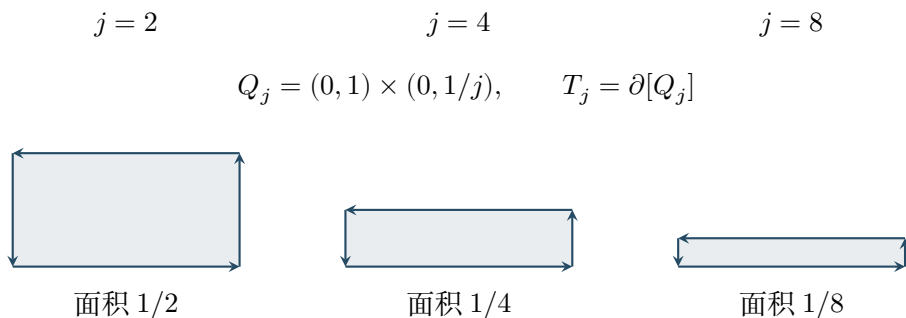
图 D.1: 薄矩形边界的平坦收敛。长边反向靠拢。质量 \mathbf{M}(T_j) = 2 + 2/j 趋于二, 而填充面积给出 \mathbb{F}(T_j) \leq 1/j , 故平坦极限为零; 有向抵消不保存无向周长。
