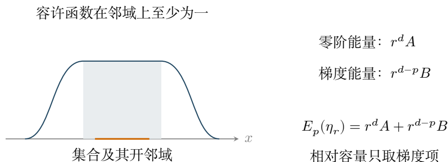
图 26.1: 容量的容许函数与过渡能量。平台与过渡区对应容许性和梯度代价。曲线只示意截断形状，容量仍是对所有容许函数及开邻域取下确界所得的量。
