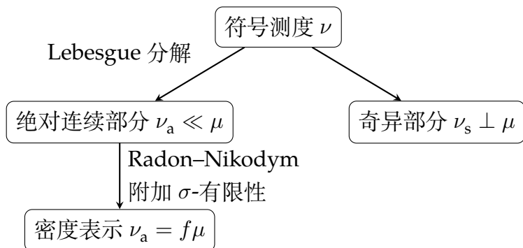
图 6.2: 测度分解的两层结构。第一层不要求参照测度 \mu 为 \sigma -有限；第二层把绝对连续部分写成密度时才使用相应假设。
