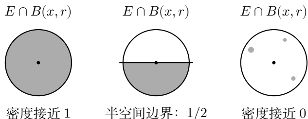
图 14.1: 局部密度。灰色表示 E 在观察球中所占的部分；三幅图分别示意占比趋近 1、保持在中间值和趋近 0 的情形。
