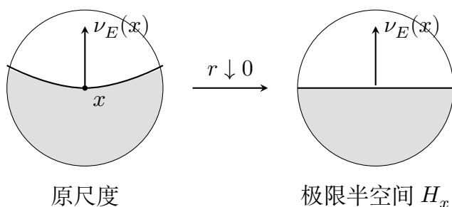
图 27.2: 约化边界的半空间缩放。灰色表示集合一侧；缩小尺度后，边界趋向 \nu_E(x)^\perp ，集合趋向相应半空间。
