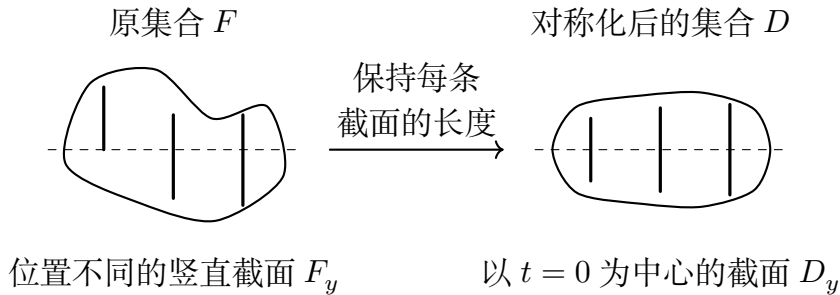
图 15.2: Steiner 对称化。图中粗线仅示意三条截面：右侧截面分别与左侧对应截面等长，但都以 t = 0 为中心。
