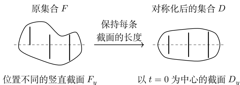
图 15.1: Steiner 对称化。图中粗线仅示意三条截面: 右侧截面分别与左侧对应截面等长, 但都以 t = 0 为中心。
