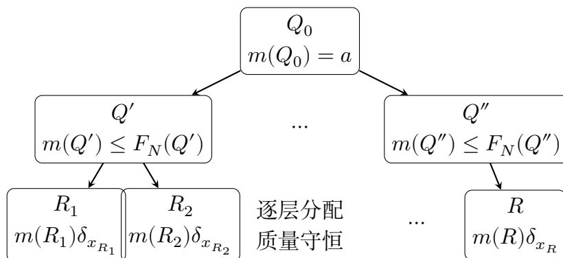
图 15.2: 二进质量分配。根质量 a 逐层向子立方体分配；每个结点受容量 F_N 控制，末层质量则变成位于 K 上的原子。图中只画出部分分支。
