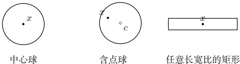
图 13.2: 三类微分基。前两类保持球形, 但观察点与球心的关系不同; 第三类若不限制长宽比, 偏心率可以任意增大。
