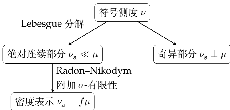
图 6.1: 测度分解的两层结构。第一层不要求参照测度 \mu 为 \sigma -有限; 第二层把绝对连续部分写成密度时才使用相应假设。
