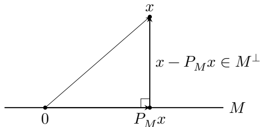
图 8.1: Hilbert 投影。向量 x 唯一分解为 M 内的最佳近似 P_M x 与正交误差 x - P_M x 。
