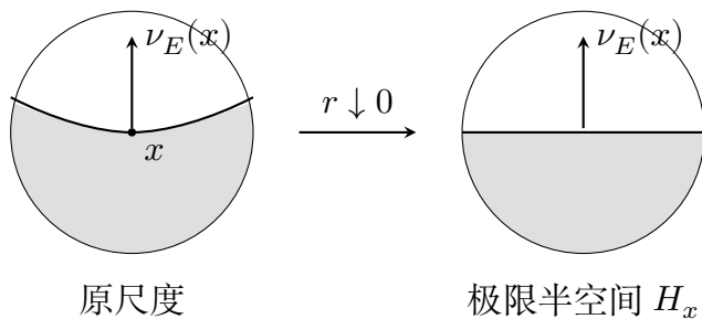
图 27.1: 约化边界的半空间缩放. 灰色表示集合一侧; 缩小尺度后, 边界趋向 \nu_E(x)^\perp , 集合趋向相应半空间.
