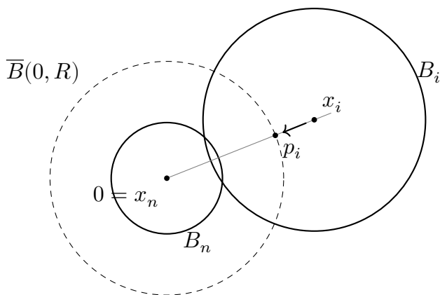
图 13.1: 径向压缩。与末球 B_n 相交的旧球中心 x_i 若位于 \overline{B}(0, R) 外，就沿射线压到 p_i ；证明的核心是这些压缩点仍有统一的分离距离。示意图不按比例。
