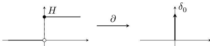
图 20.1: 跳跃的分布导数。Heaviside 函数的变化集中在原点, 故 \partial T_H = \delta_0 。
