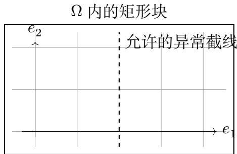
图 21.1: ACL 坐标截线。实线示意良好截线, 虚线只表示某个允许排除的截线; 真正的例外族由横向零测集参数化。
