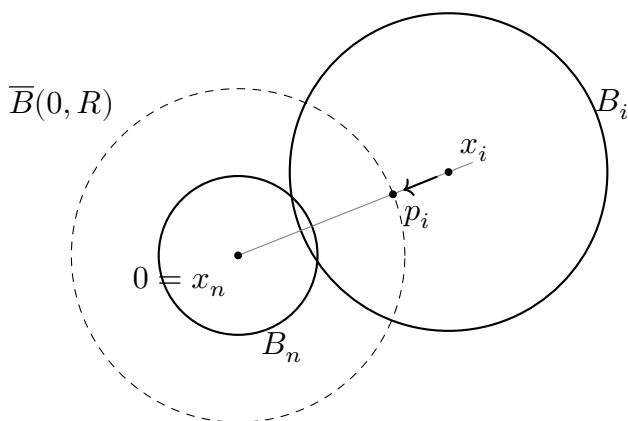
图 13.1: Besicovitch 几何引理中的径向压缩: 与末球 B_n 相交的旧球中心 x_i 若位于 \overline{B}(0, R) 外, 就沿射线压到 p_i ; 证明的核心是这些压缩点仍有统一的分离距离。示意图不按比例。
