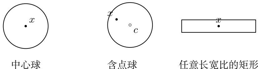
图 13.2: 微分基中三类允许集合的几何差别。前两类保持球形，但观察点与球心的关系不同；第三类若不限长宽比，偏心率可以任意增大。
