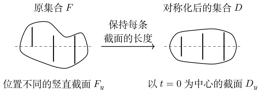
图 15.1: 沿末坐标方向的 Steiner 对称化. 图中粗线仅示意三条截面: 右侧截面分别与左侧对应截面等长, 但都以 t = 0 为中心.
