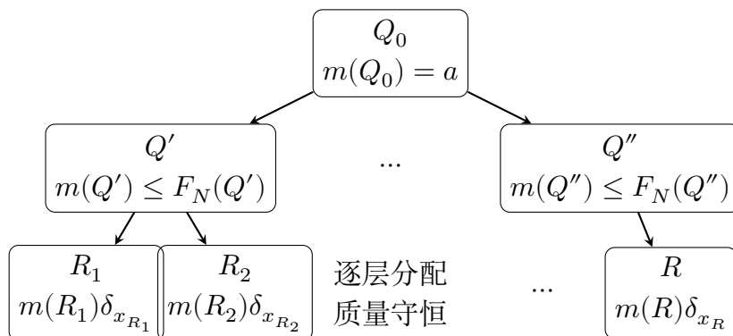
图 15.2: Frostman 构造中的有限二进立方体树。根质量 a 逐层向子立方体分配；每个结点受容量 F_N 控制，末层质量则变成位于 K 上的原子。图中只画出部分分支。
