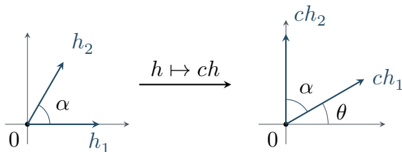
图 1.1: 复线性微分的旋转与伸缩. 图中取 \theta = \pi/6 、 \rho > 1 , 相交方向的有向夹角 \alpha 不变。
