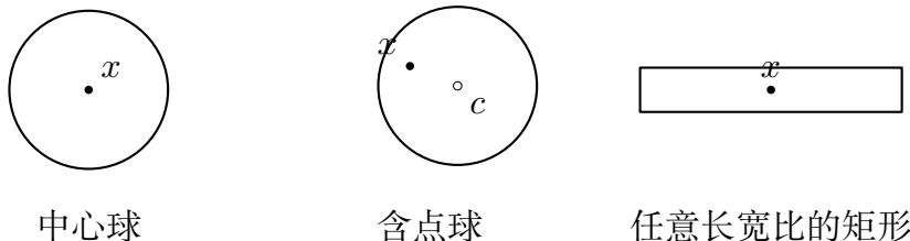
图 13.2: 微分基中三类允许集合的几何差别。前两类保持球形，但观察点与球心的关系不同；第三类若不限长宽比，偏心率可以任意增大。
