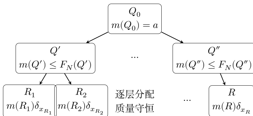
图 15.3: 二进质量分配。根质量 a 逐层向子立方体分配; 每个结点受容量 F_N 控制, 末层质量则变成位于 K 上的原子。图中只画出部分分支。
