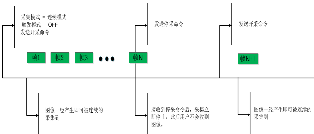
图 3-13 非触发+连续采集模式
