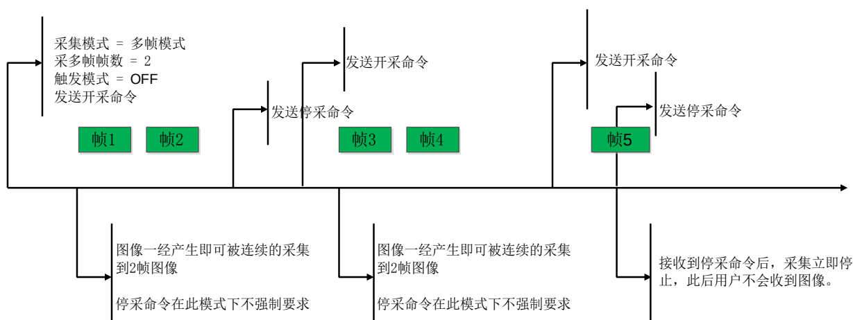
图 3-15 非触发+多帧模式
