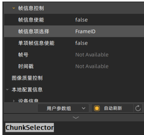
图 3-25 U3 帧信息节点
