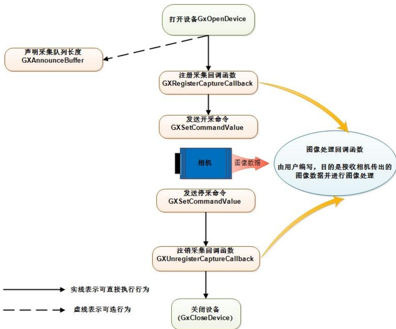
图 1-5 回调采集流程
