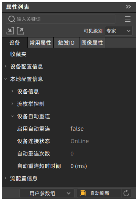
图 2-22 自动重连属性节点
