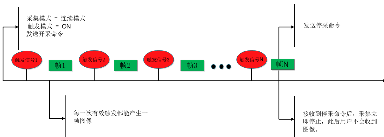
图 3-14 触发+连续采集模式
