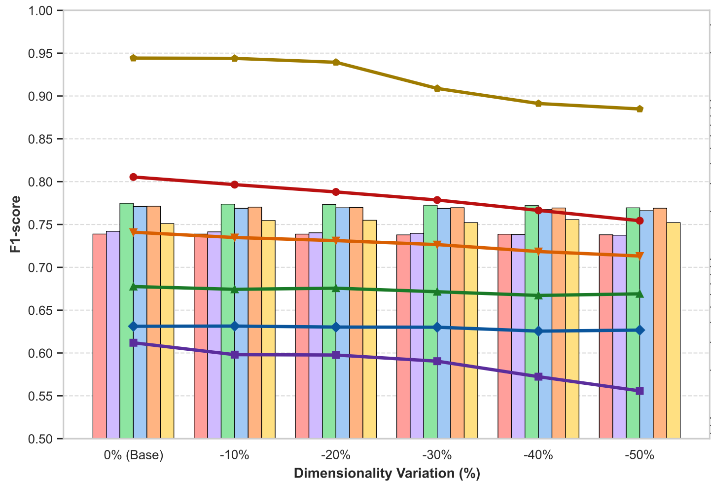
Dataset: Bondora
