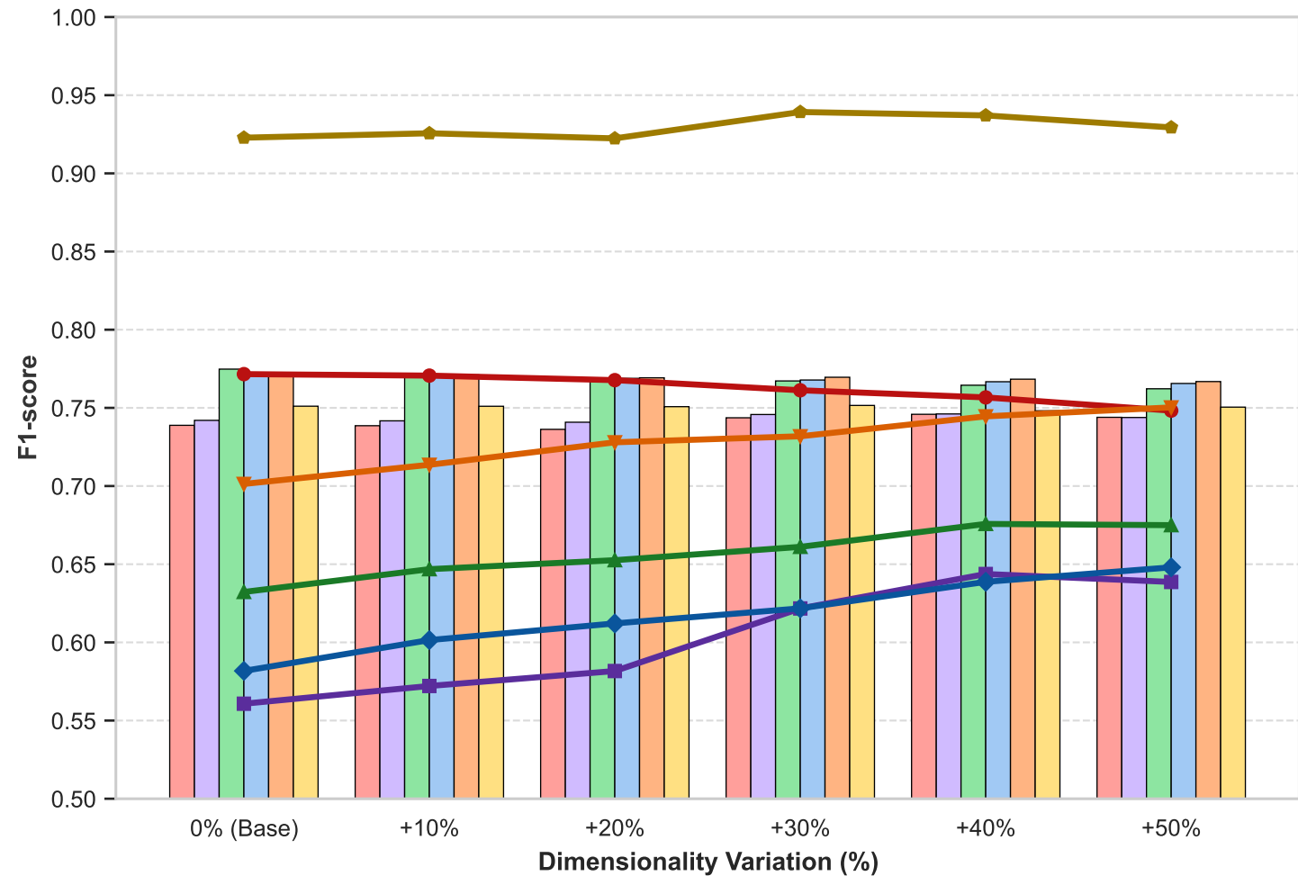
Dataset: Bondora
