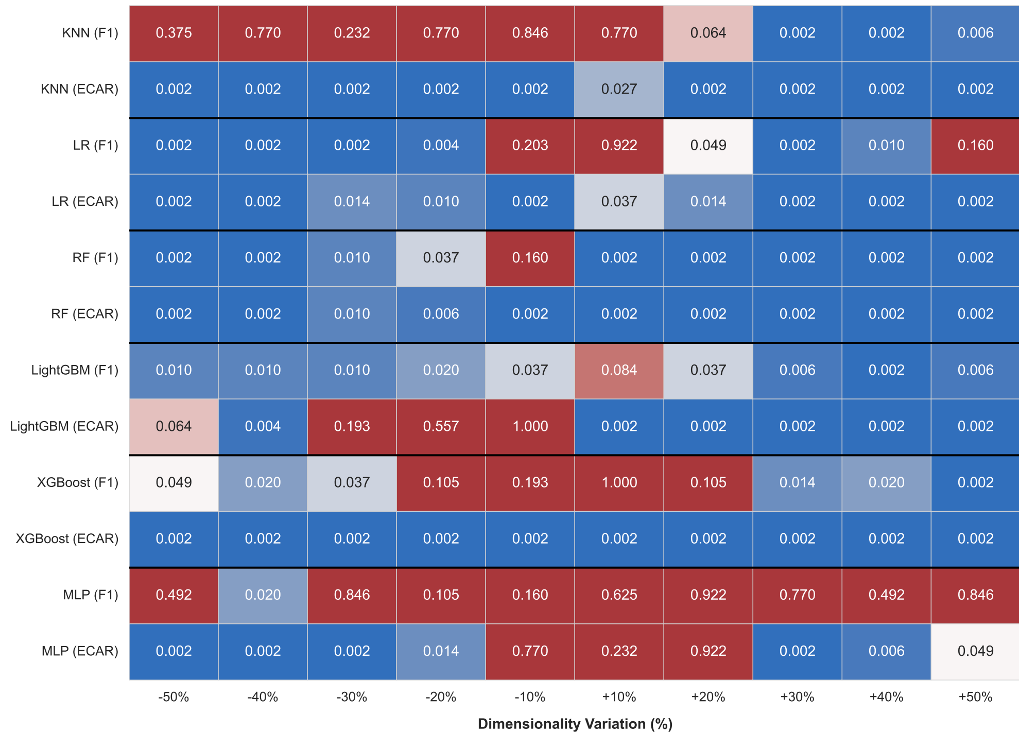
Dataset: Bondora
