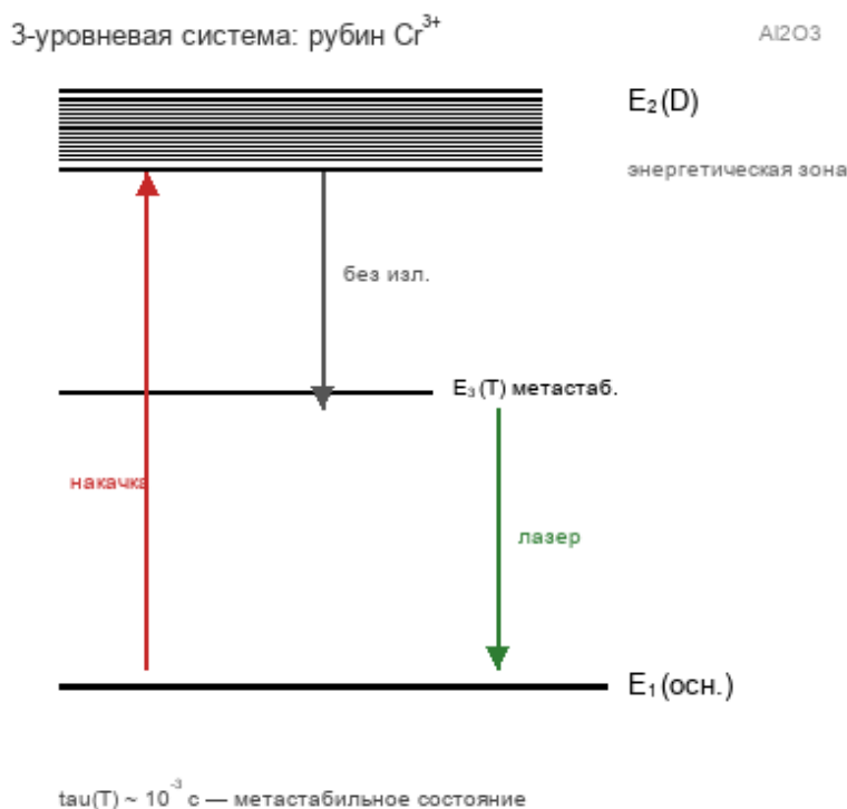
Рис. 3.4. Трёхуровневая схема рубинового лазера (ионы Cr 3+ )
