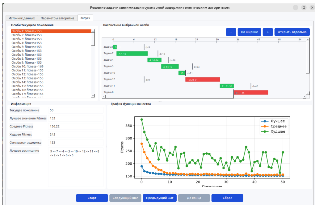
Рисунок 3 — Вкладка «Запуск»
