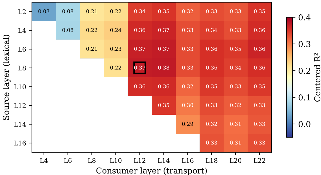
Figure 5: Deposit map R^2 across layer pairs (subj→verb)
