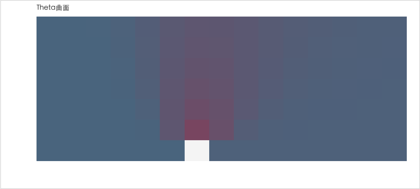
Theta曲面数据（第1组）
