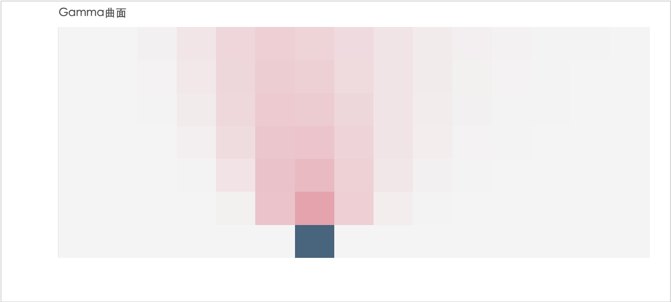
Gamma曲面数据（第1组）
