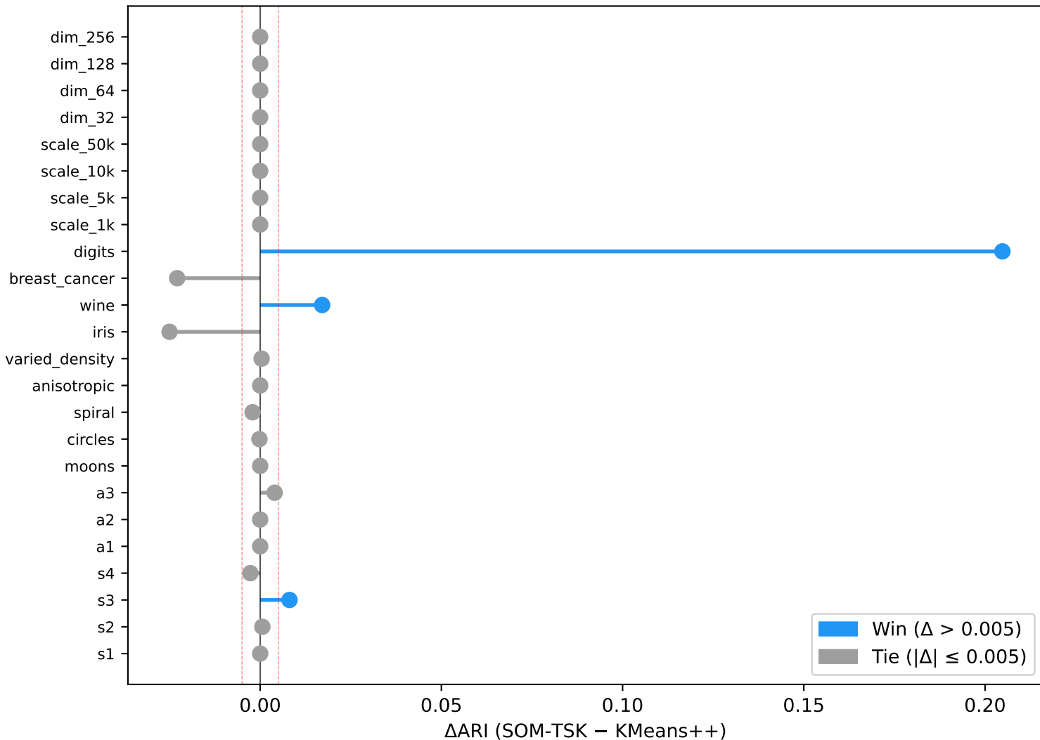
ARI Improvement per Dataset
