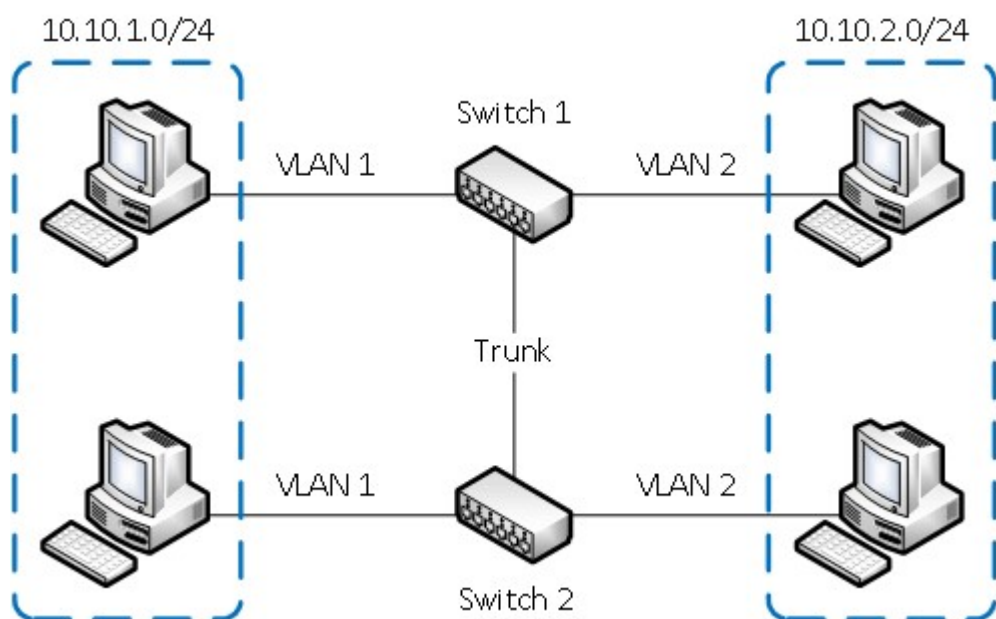
Рисунок 2. Объединение в единую сеть компьютеров, подключенных к разным коммутаторам
