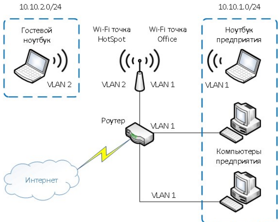
Рисунок 4. Разделение гостевой Wi-Fi сети и Wi-Fi сети предприятия при помощи VLAN
