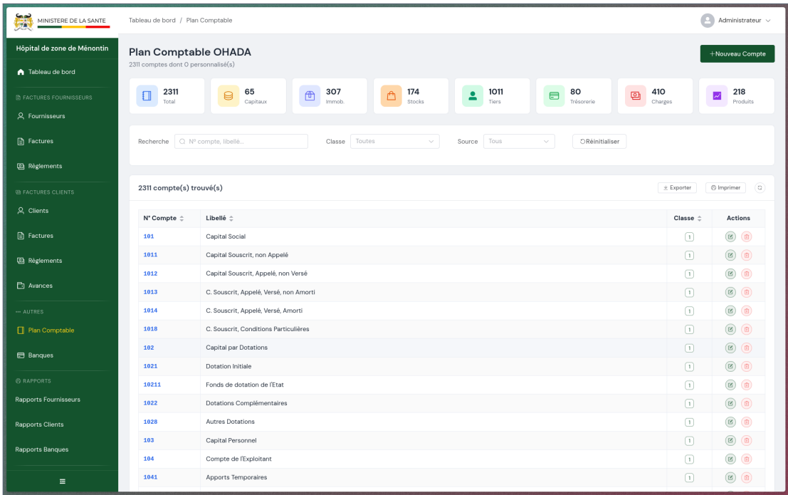
Figure 3.13 – Consultation du plan comptable OHADA.
