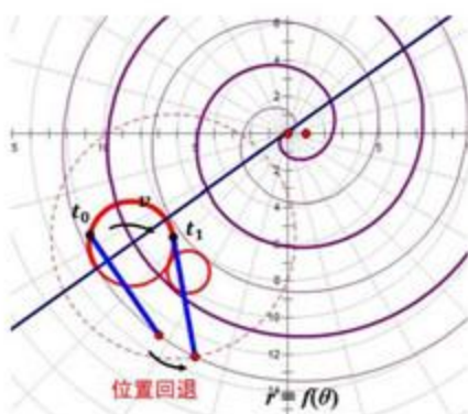
图 26 龙头盘旋方向约束示意图
