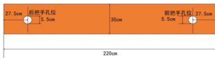
图 1.2: 龙身、龙尾俯视数据图
