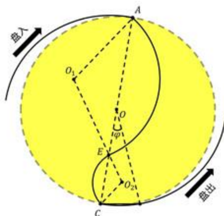
图 4.19: 情况四判断角示意图
