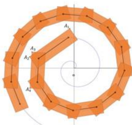
图 2.6: 板凳龙盘入示意图 (橙色矩形为板凳)
