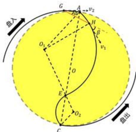
图 4.25: 速度迭代示意图
