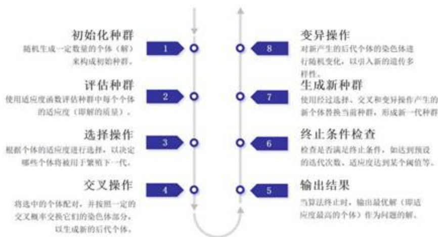
图8 遗传算法的具体步骤
