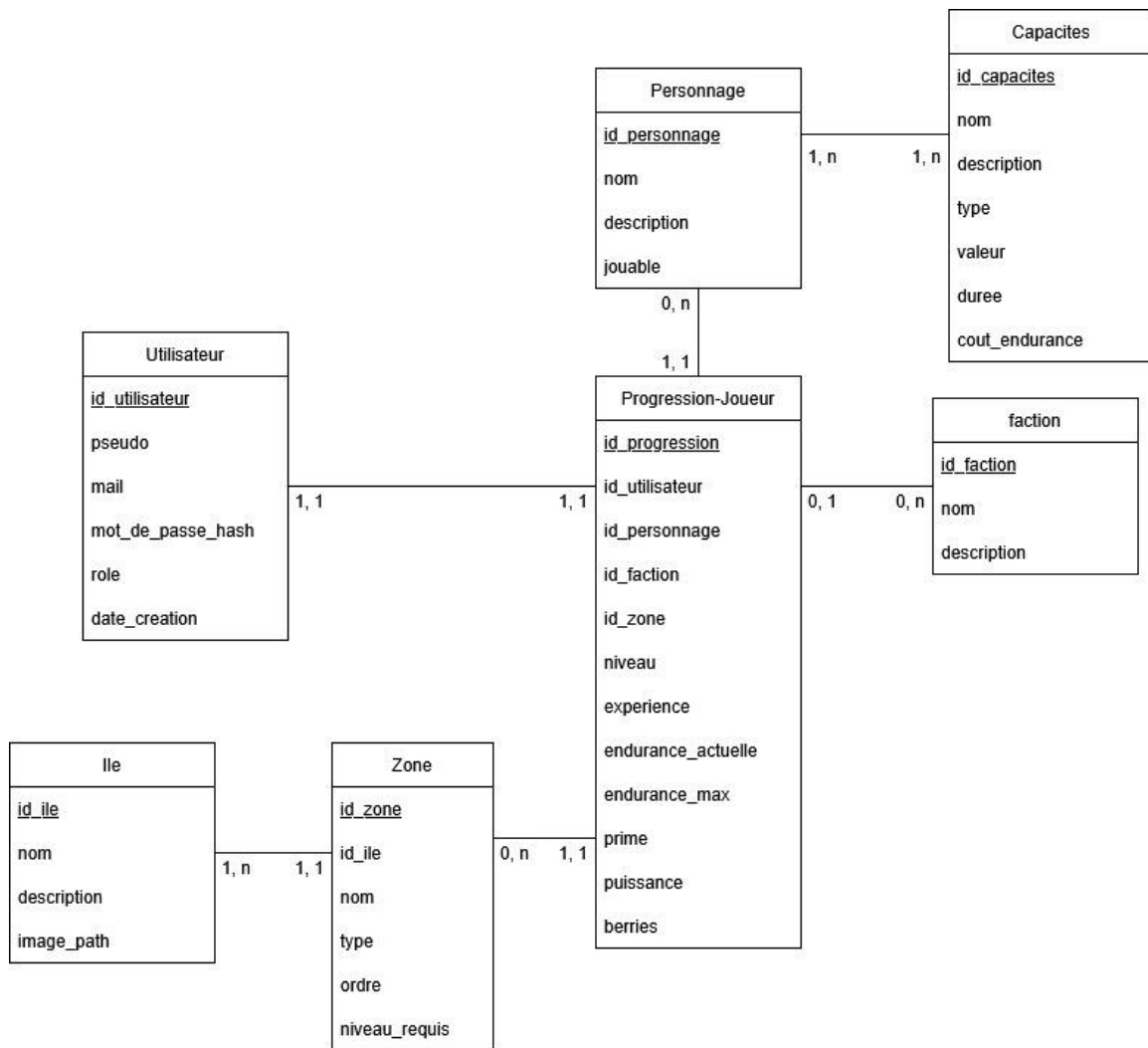
Figure 6 : Modèle Conceptuel de Données de l'application One Piece RPG
