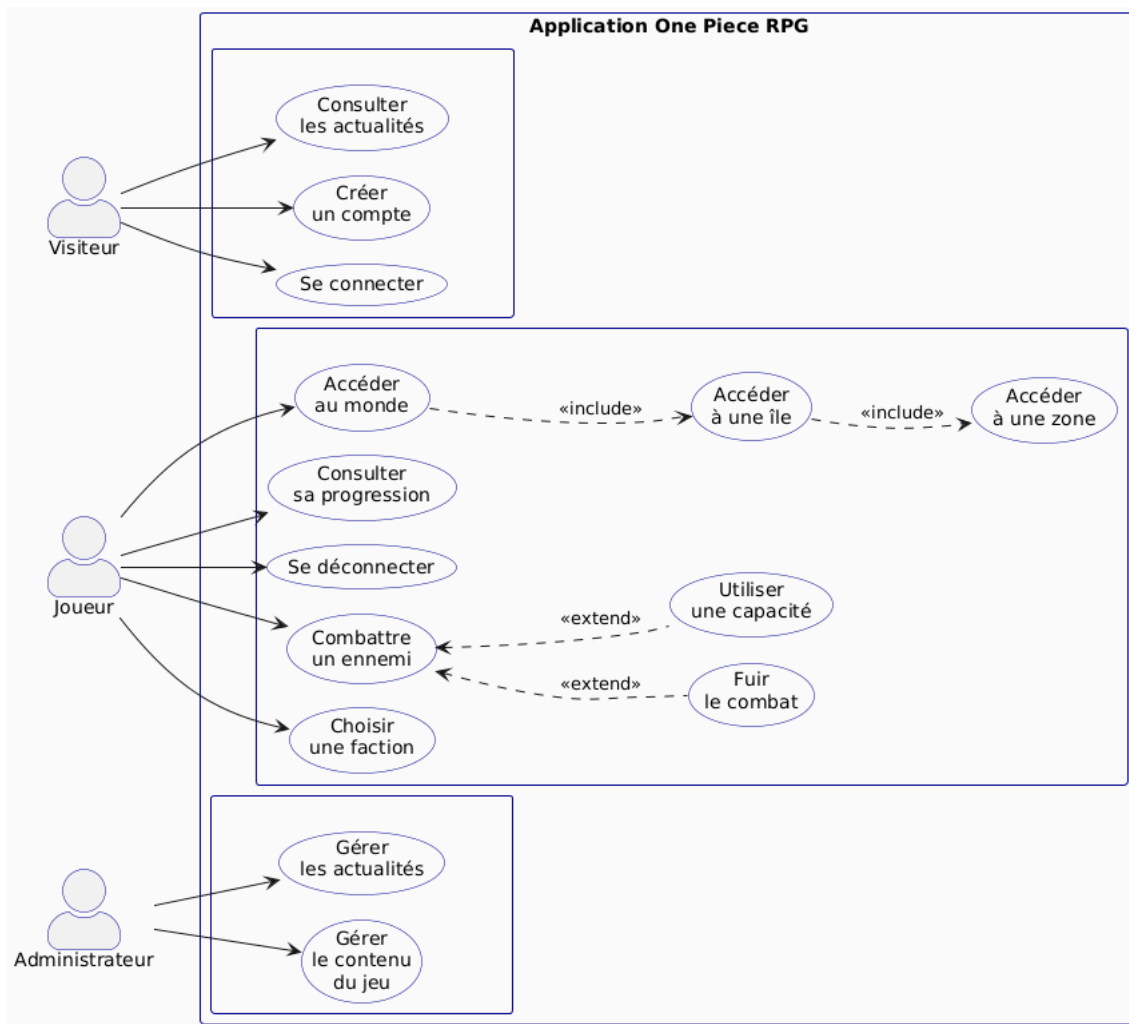
Figure 2 : Diagramme de cas d'utilisation de l'application One Piece RPG
