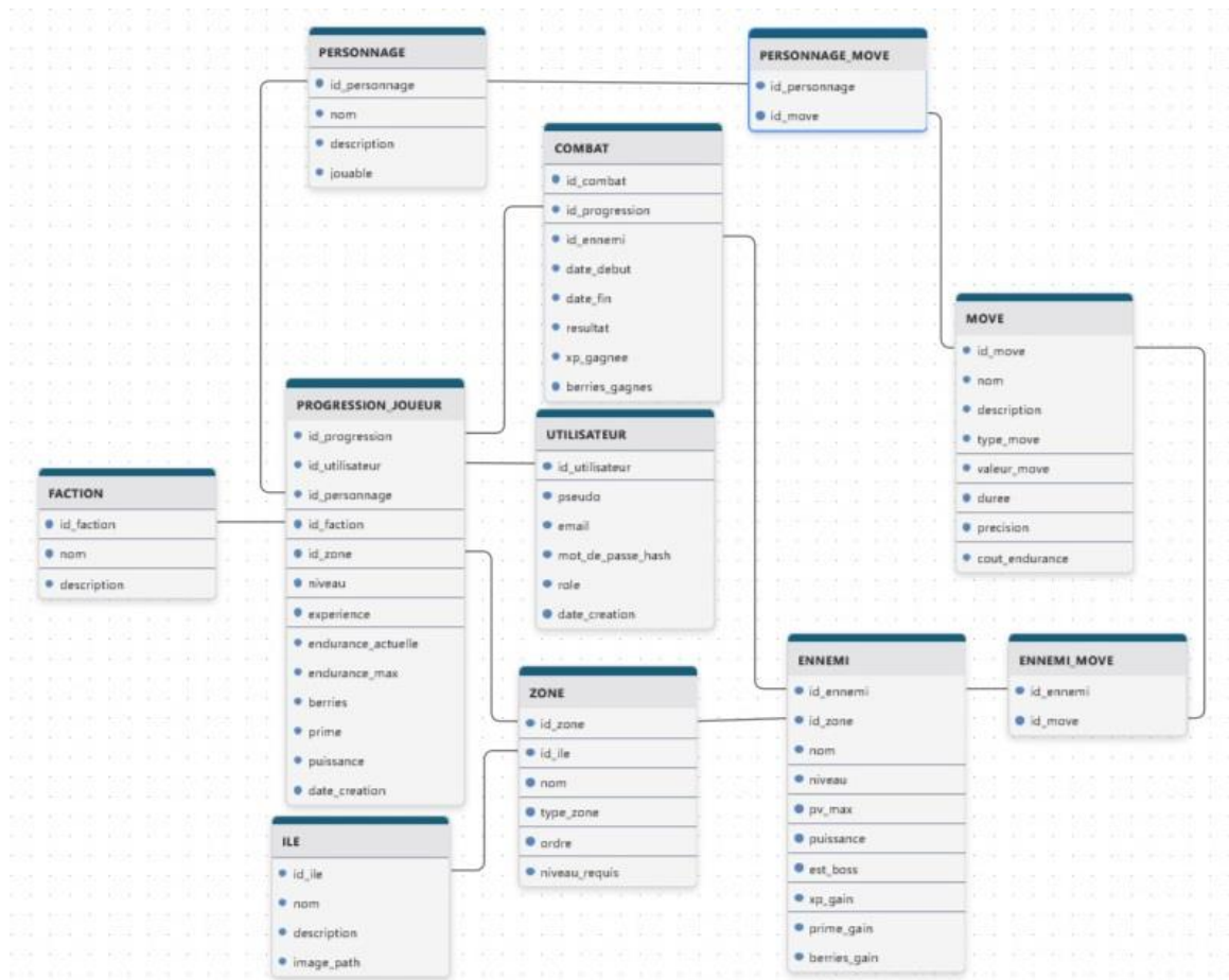
Figure 7 : Modèle Physique de données de l'application One Piece RPG
