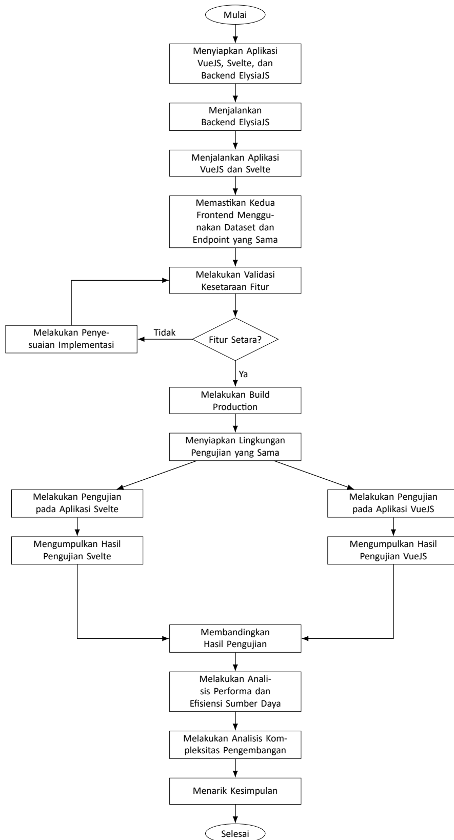
Gambar 3.1 Flowchart Tahapan Skripsi
