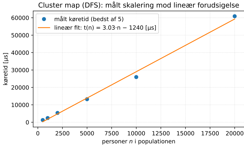
Figure 4: Målt køretid for klusterkort-konstruktionen (DFS) vha. time.perf_counter , bedst af 5 gentagelser pr. punkt. Den lineære fit t(n) \approx c \cdot n bekræfter kompleksitetsanalysen T = \Theta(n + m) = \Theta(n) fra §4.1 (invariant I1 giver m \leq 2n ).
