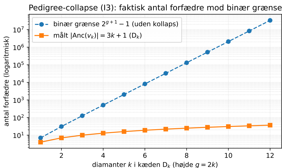
Figure 3: Pedigree-collapse i tal: for diamanatkæden D_k er det faktiske antal forfædre |\text{Anc}(v_k)| = 3k + 1 , mens den naive binære grænse 2^{g+1} - 1 vokser eksponentielt med højden g = 2k . Målt med programmets ancestors_iterative .
