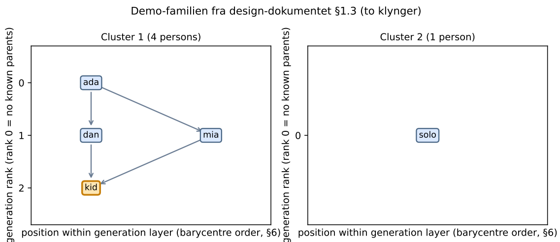
Figure 1: Demo-familien fra design-dokumentet §1.3 tegnet af programmets eget view-modul. To klynger: sammenbrudsfamilien til venstre (ada er både mias og dans far, hvilket er pedigree-collapse, invariant I3 ) og den isolerede person solo til højre. Søgeudgangspunktet kid er fremhævet.
