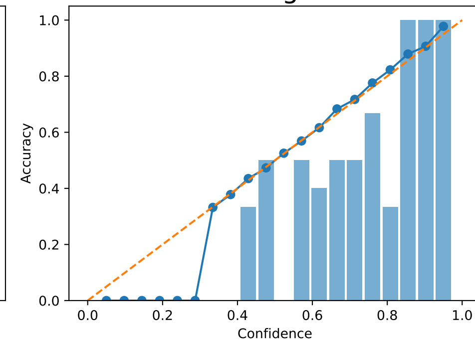
DPO - Forget 1 %
