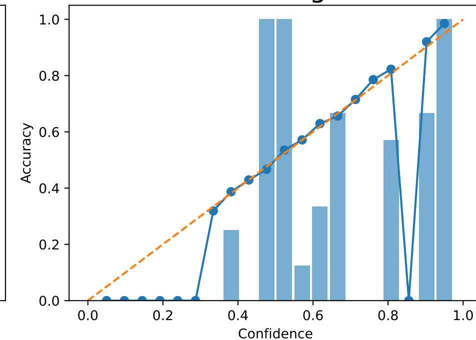
NPO - Forget 1 %
