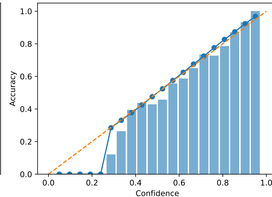
NPO - Retain 99%
