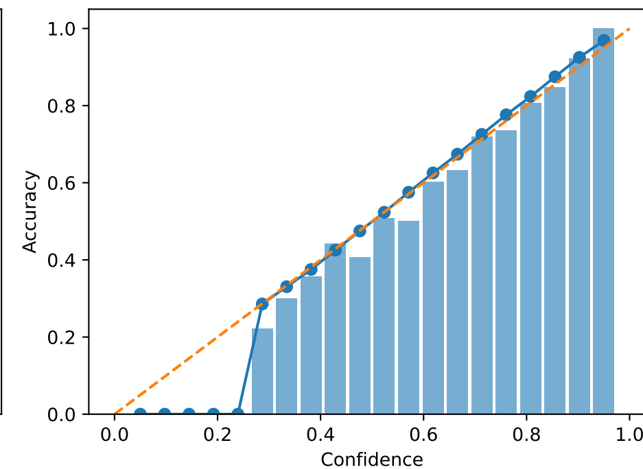
DPO - Retain 99%
