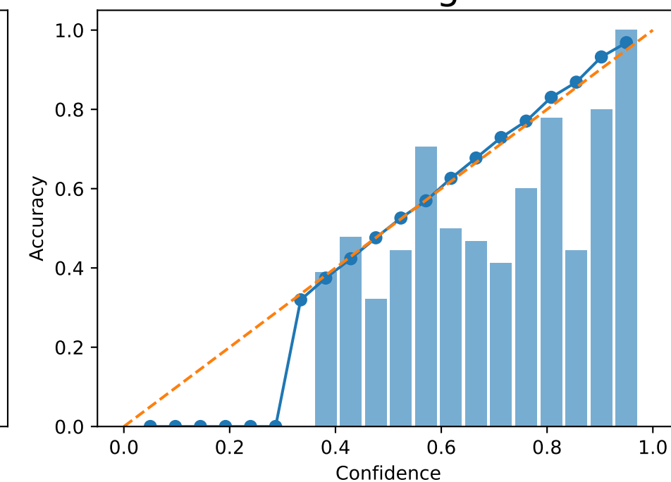
NPO - Forget 5 %
