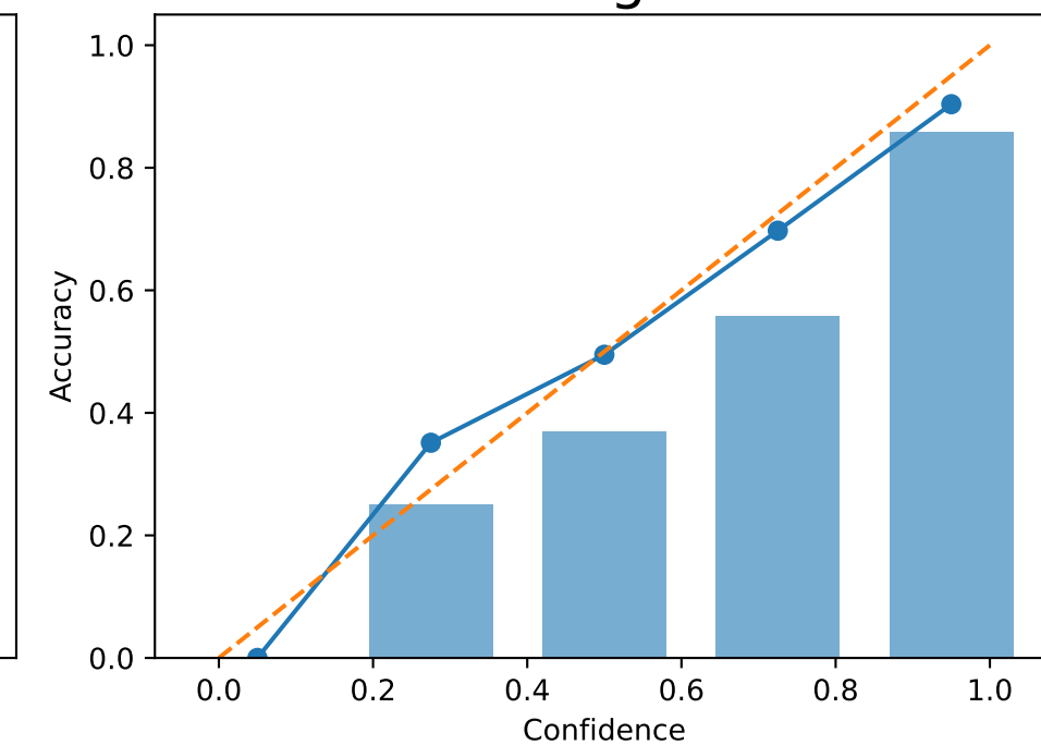
DPO - Forget 10 %
