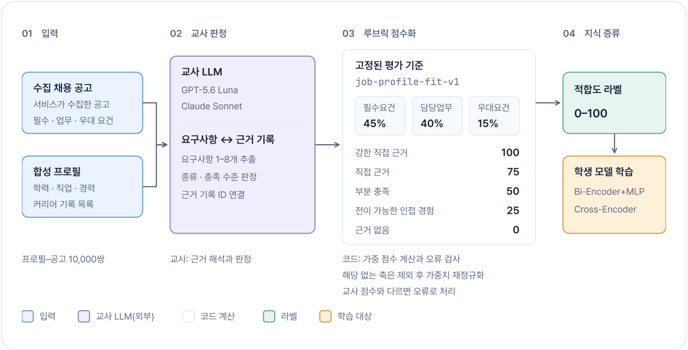
그림 3.3 루브릭 기반 교사 지식 종류의 적합도 라벨 생성 과정
