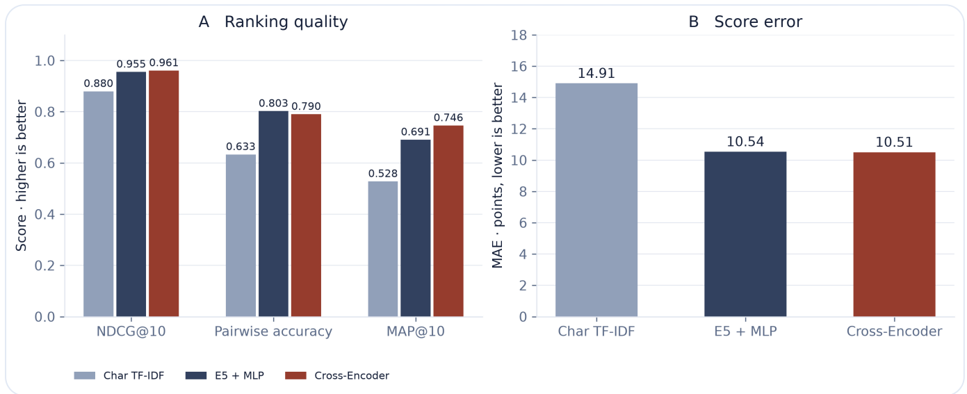
그림 9.1 모델별 순위 품질과 점수 오차 (평가 분할)
