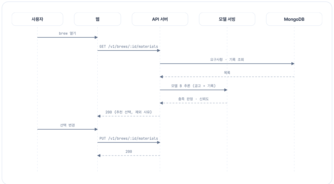
그림 6.2.8 포트폴리오 재료 선정 기능의 시퀀스 다이어그램
