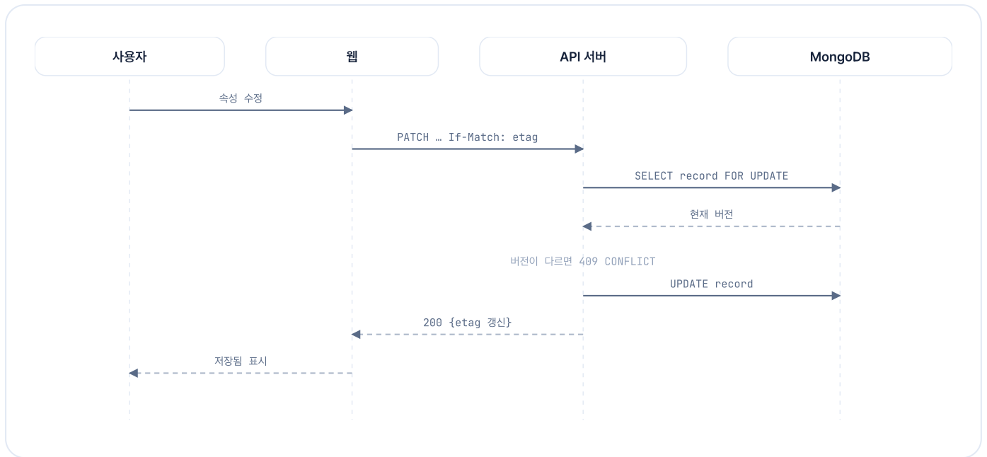
그림 6.2.3 기록 속성 편집 기능의 시퀀스 다이어그램
