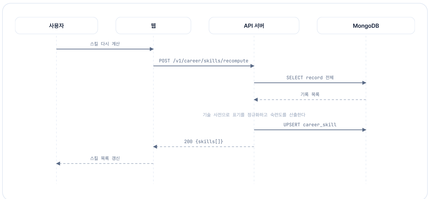
그림 6.2.4 스킬 자동 집계 기능의 시퀀스 다이어그램
