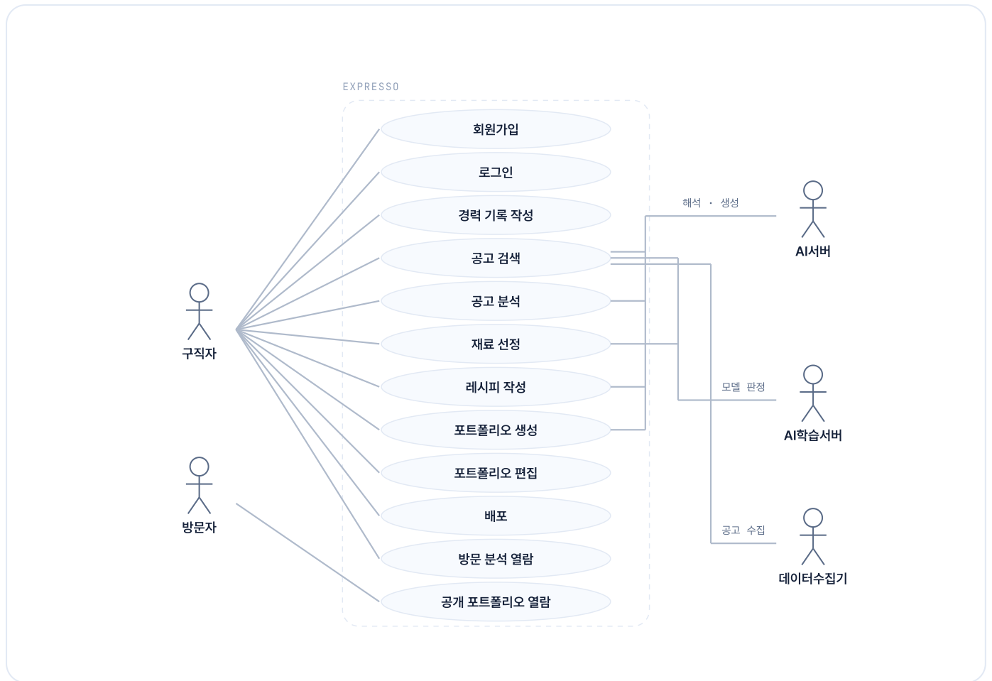
그림 2.2 사용자용 유스케이스 다이어그램
