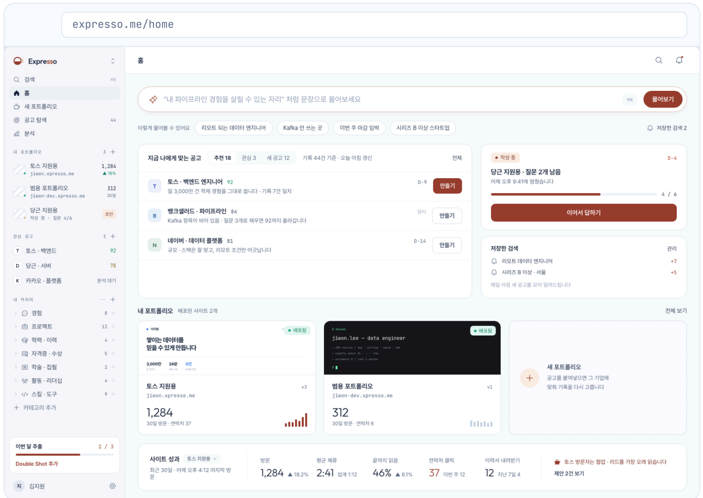
그림 5.3.1 Home (화면번호 00)
