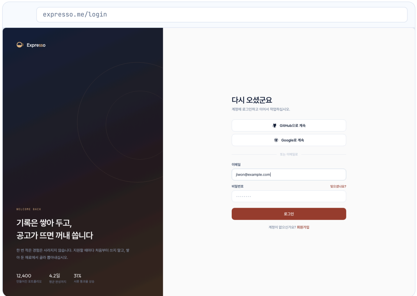
그림 5.3.25 로그인 (화면번호 10)
