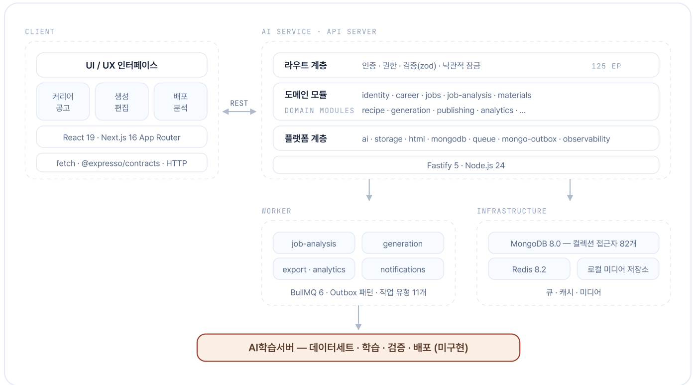
그림 6.1 시스템 아키텍처
