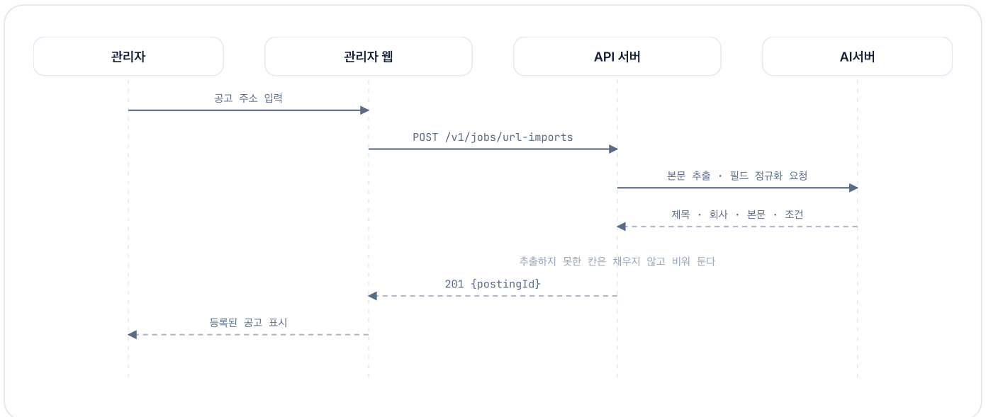
그림 6.3.4 URL로 공고 가져오기 기능의 시퀀스 다이어그램
