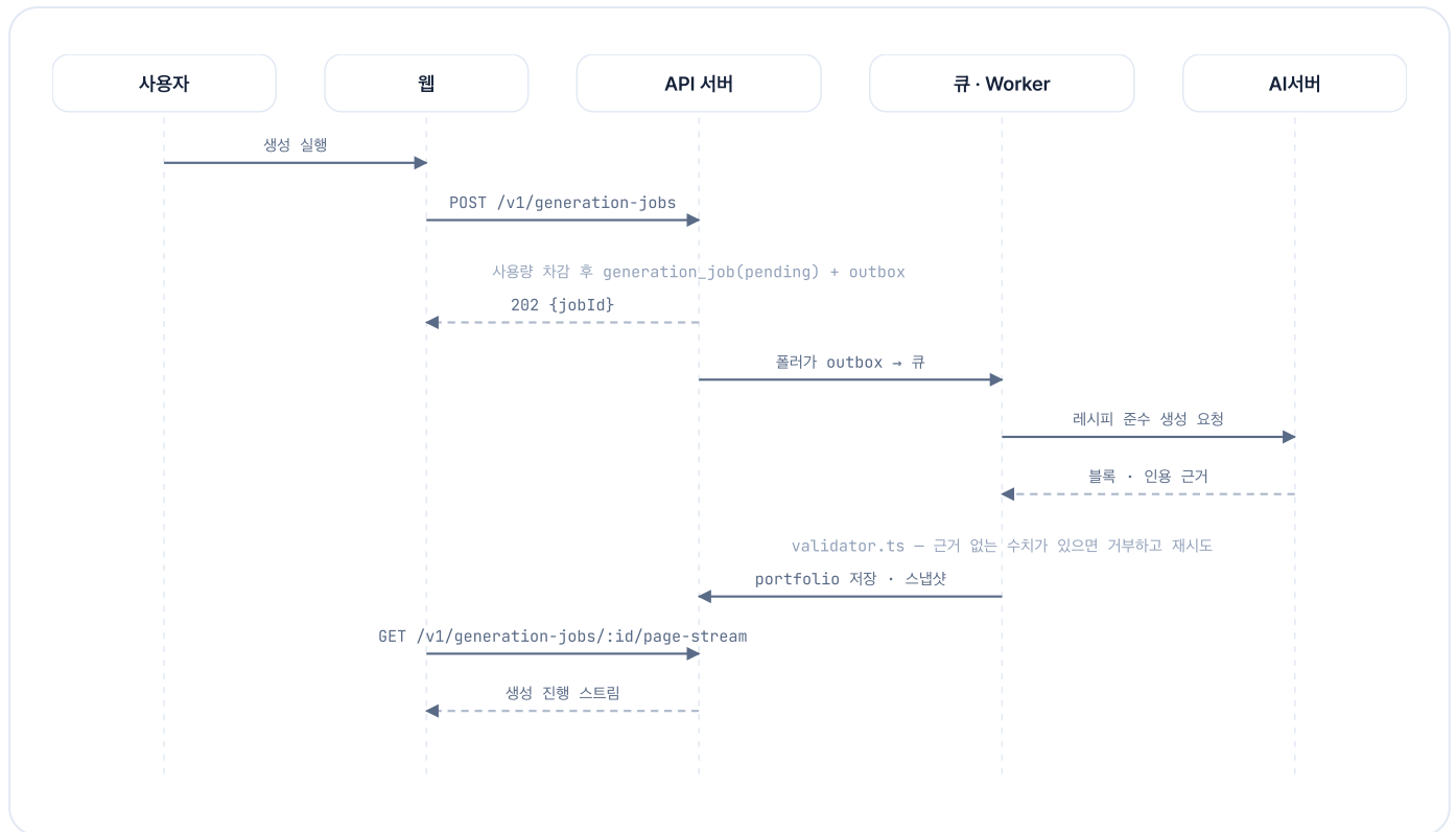
그림 6.2.11 포트폴리오 생성 실행 기능의 시퀀스 다이어그램
