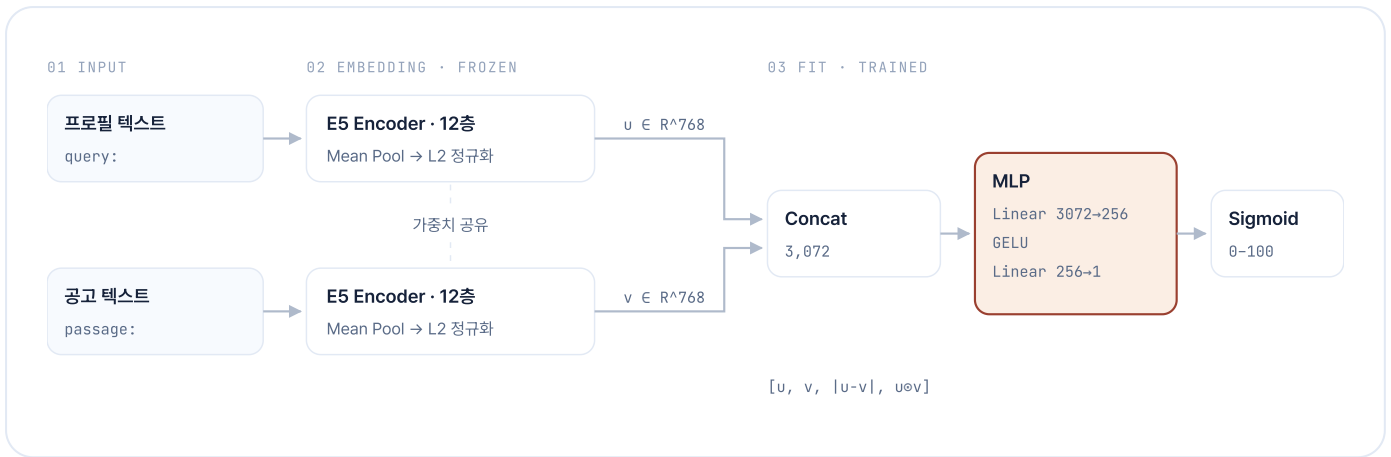
그림 4.2 Bi-Encoder+MLP 적합도 모델의 구조
