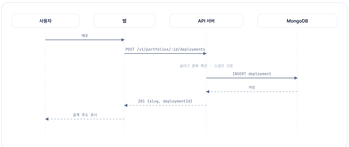
그림 6.2.13 배포와 주소 발급 기능의 시퀀스 다이어그램
