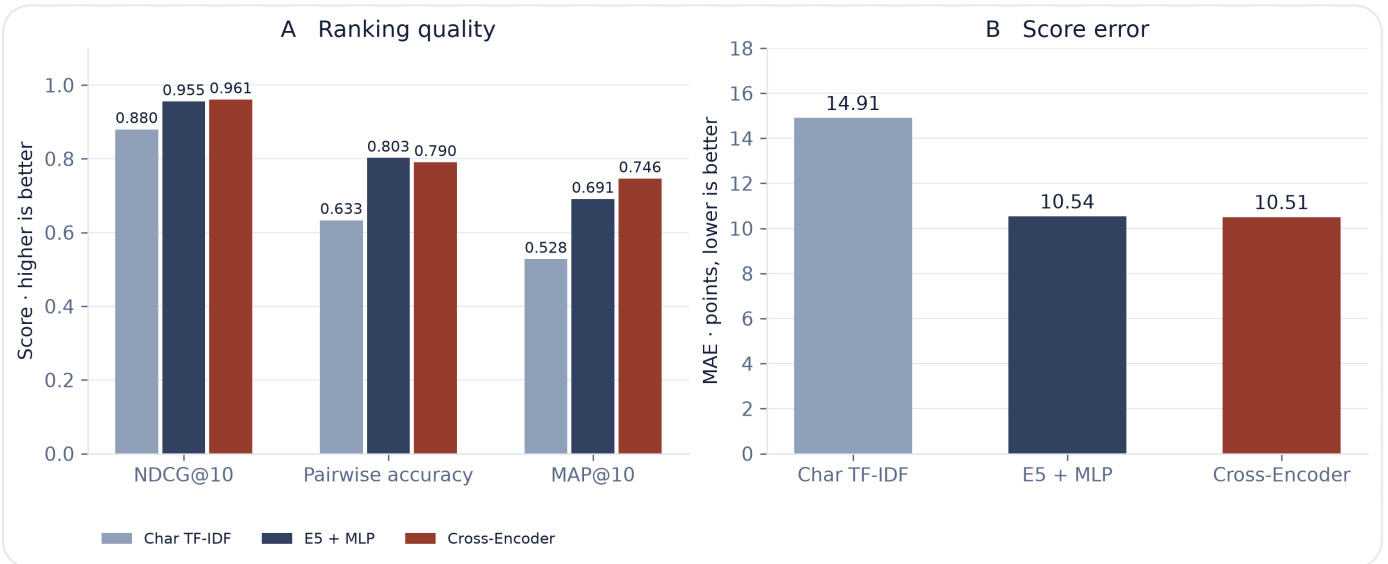
그림 9.1 모델별 순위 품질과 점수 오차 (평가 분할)
