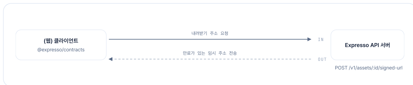
그림 7.3.9 자산 서명 URL 발급의 요청·응답 방향
