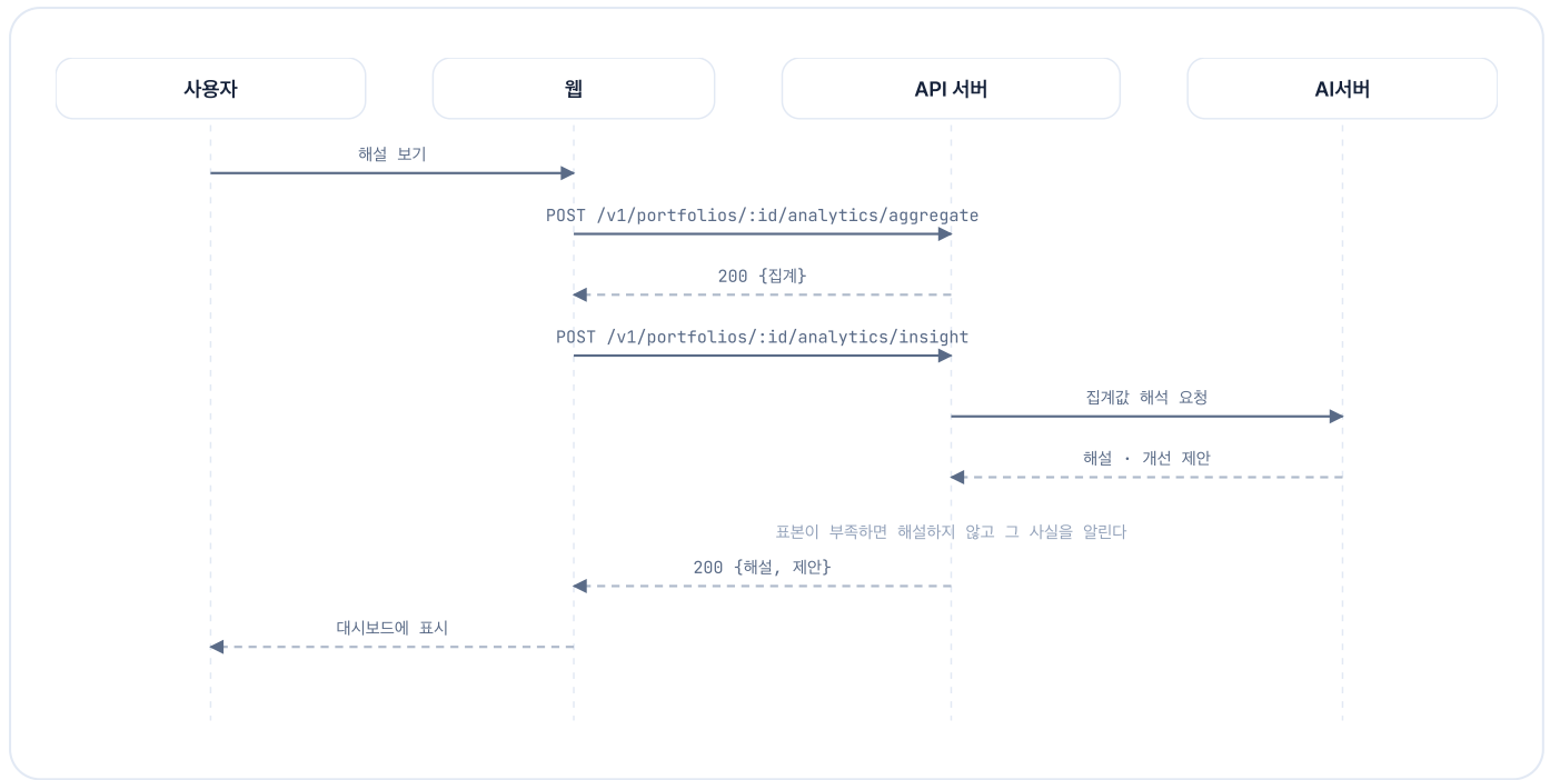
그림 6.2.16 읽기 패턴 해설 기능의 시퀀스 다이어그램
