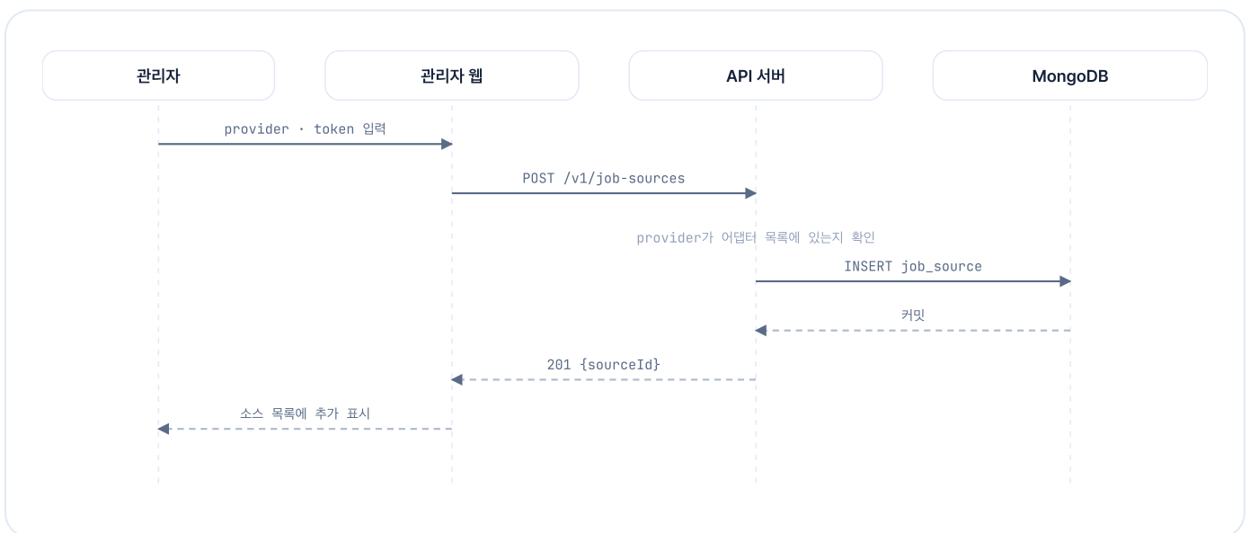
그림 6.3.2 수집 소스 등록 기능의 시퀀스 다이어그램
