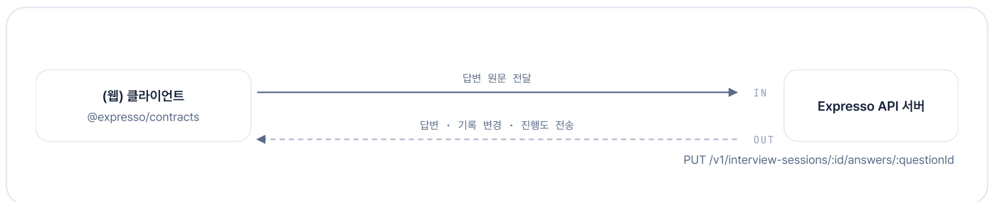
그림 7.3.18 인터뷰 답변 저장의 요청 · 응답 방향
