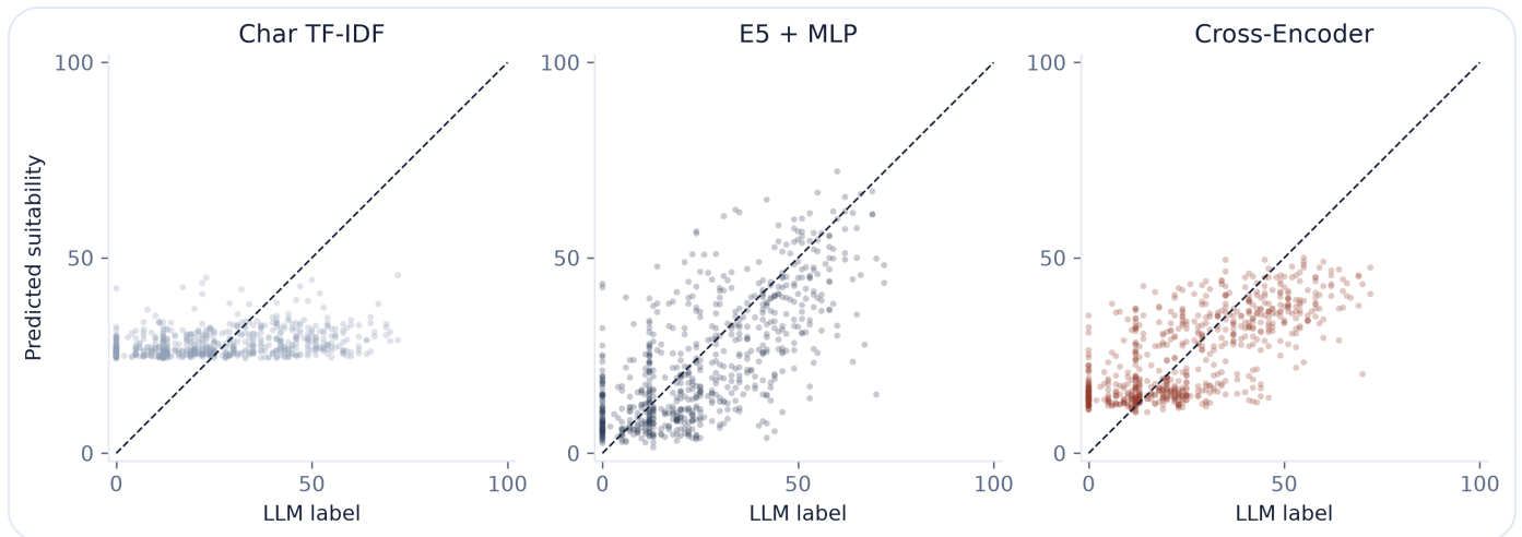
그림 9.2 LLM 라벨과 모델 예측값 (평가 분할 700쌍)
