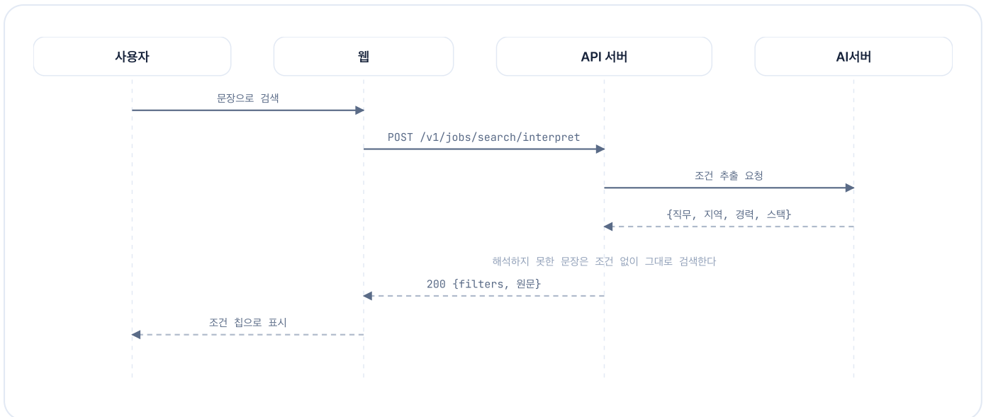
그림 6.2.5 자연어 검색 조건 변환 기능의 시퀀스 다이어그램
