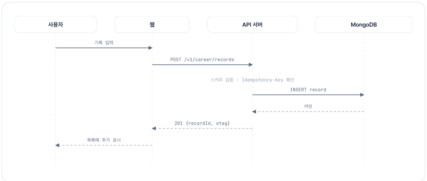
그림 6.2.2 기록 직접 만들기 기능의 시퀀스 다이어그램
