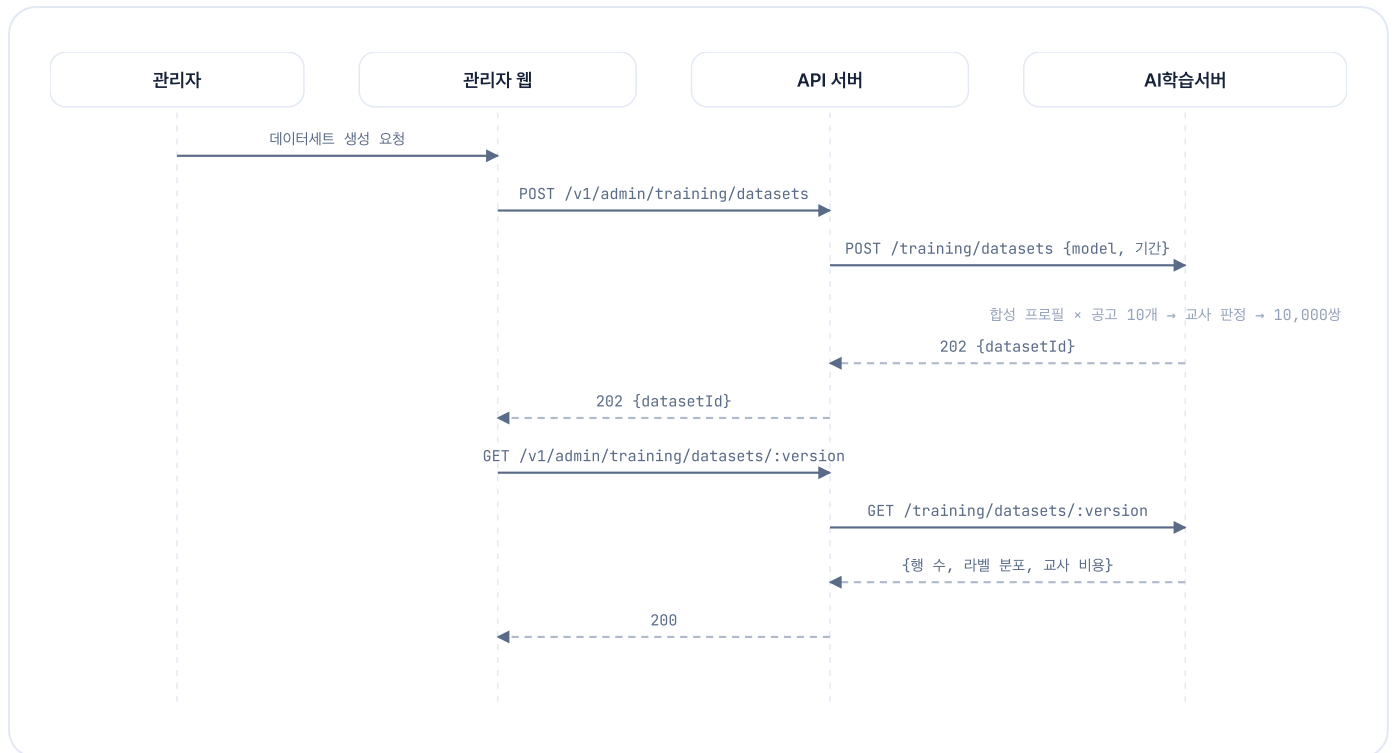
그림 6.3.7 학습 데이터세트 생성 기능의 시퀀스 다이어그램
