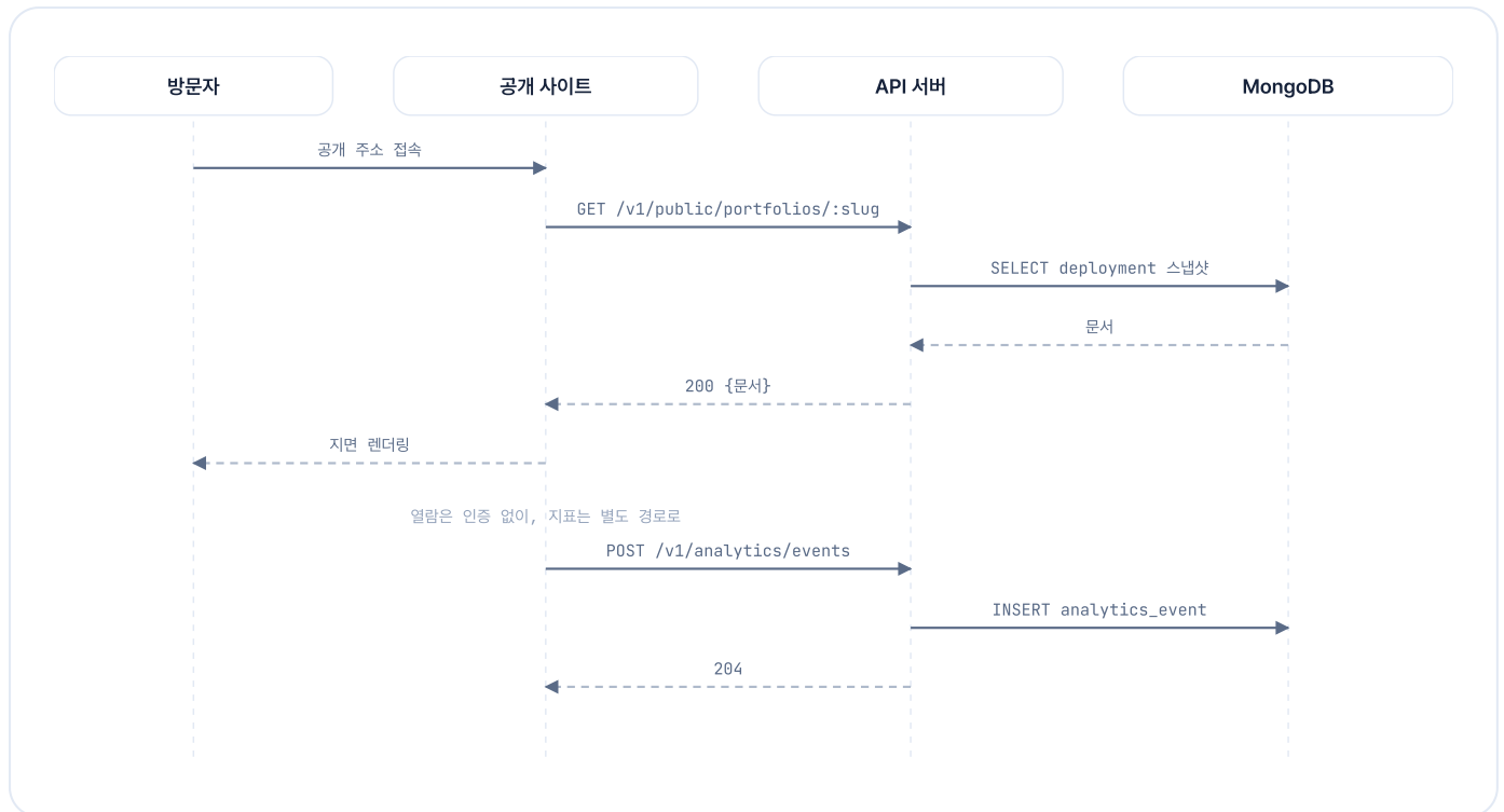
그림 6.2.15 방문 지표 수집 기능의 시퀀스 다이어그램
