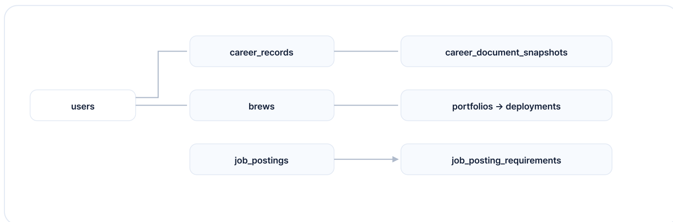
그림 8.1 핵심 컬렉션의 참조 관계. 화살표는 문서의 식별자 참조를 뜻한다.
