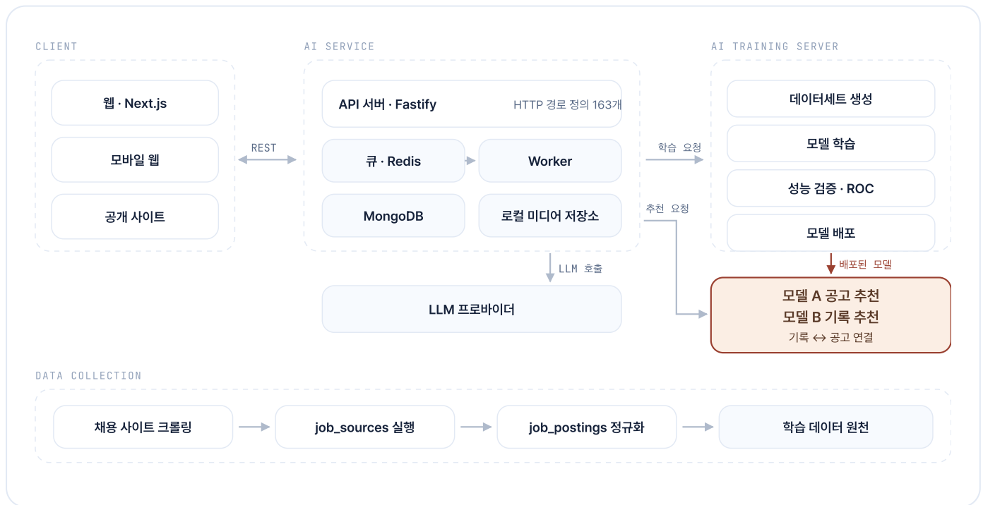
그림 2.2 서비스 시나리오 구성도
