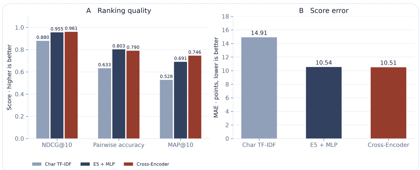
그림 9.2 모델별 순위 품질과 점수 오차 (평가 분할)
