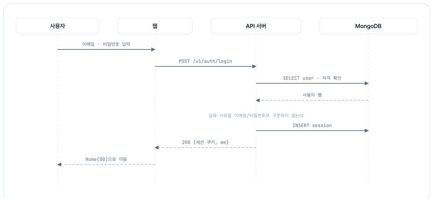
그림 6.2.1 로그인 기능의 시퀀스 다이어그램
