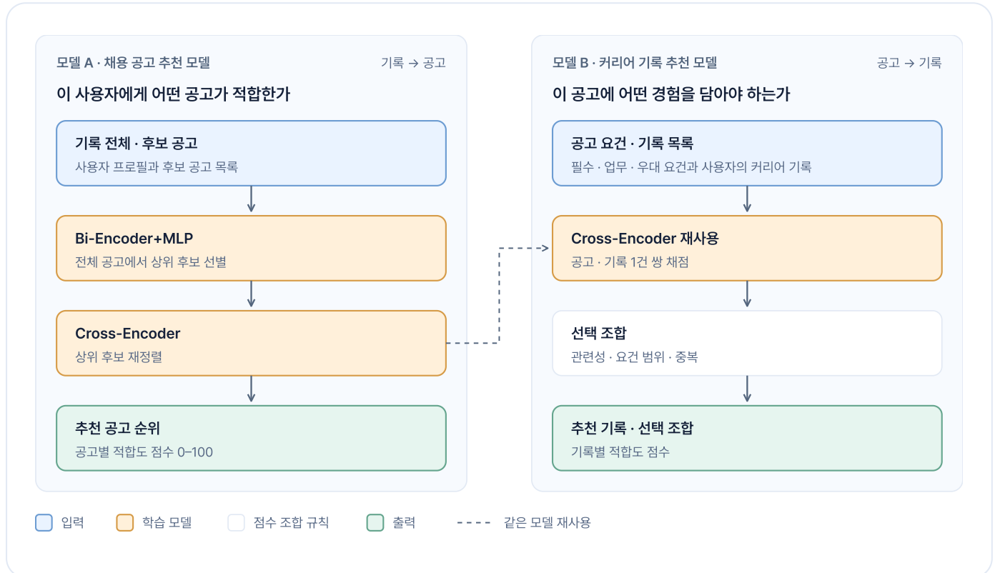
그림 3.1 채용 공고 추천 모델과 커리어 기록 추천 모델의 구성
