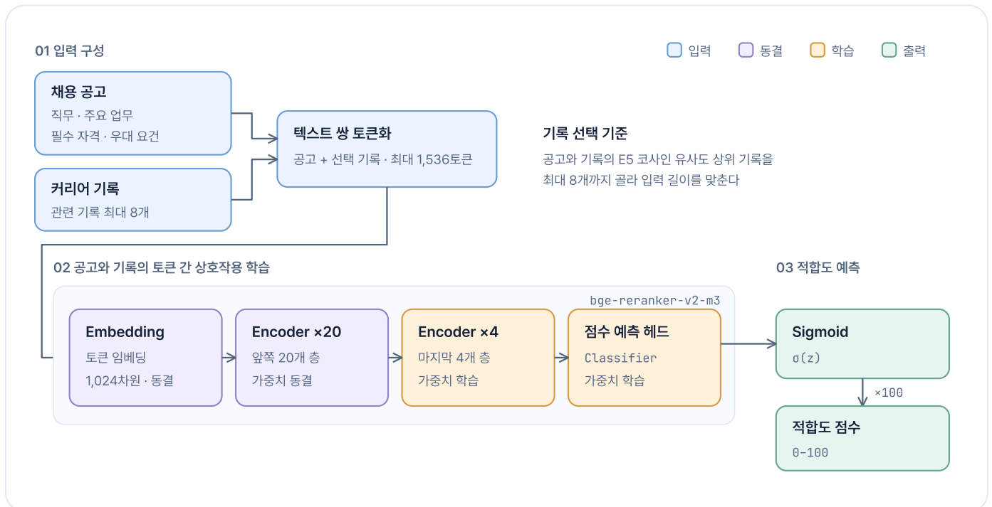
그림 4.3 Cross-Encoder 적합도 모델의 구조
