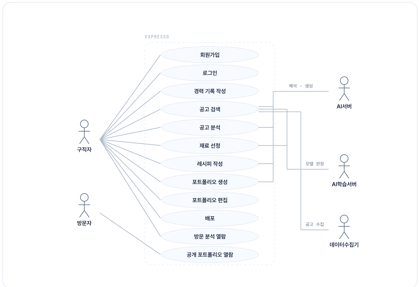
그림 2.3 사용자용 유스케이스 다이어그램
