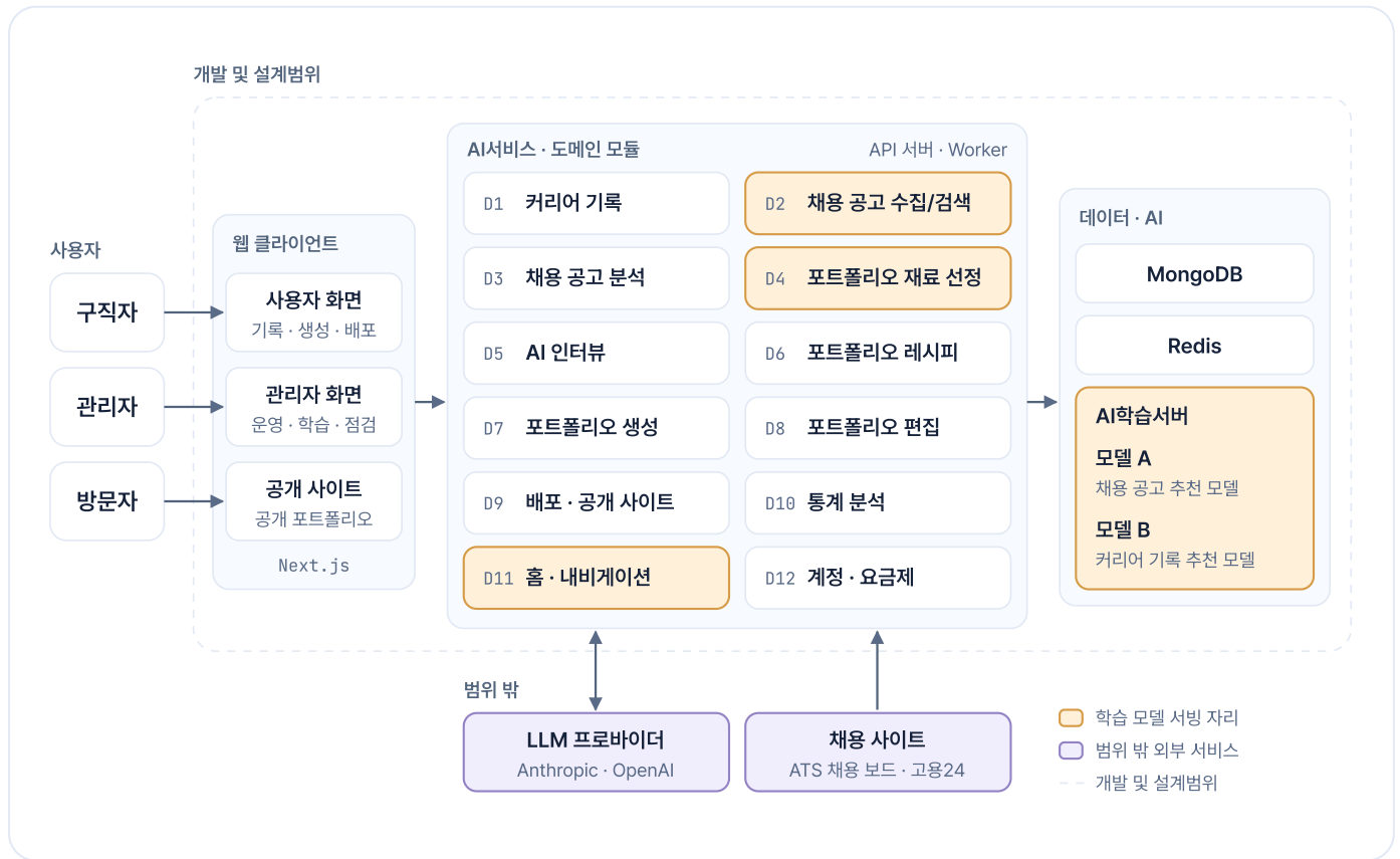
그림 1.2 서비스의 전체 구성과 설계범위
