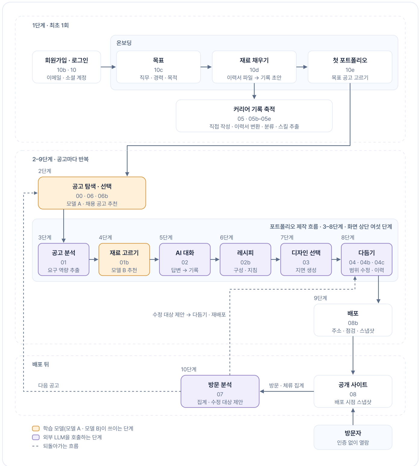
그림 2.1 전체 사용자 플로우
