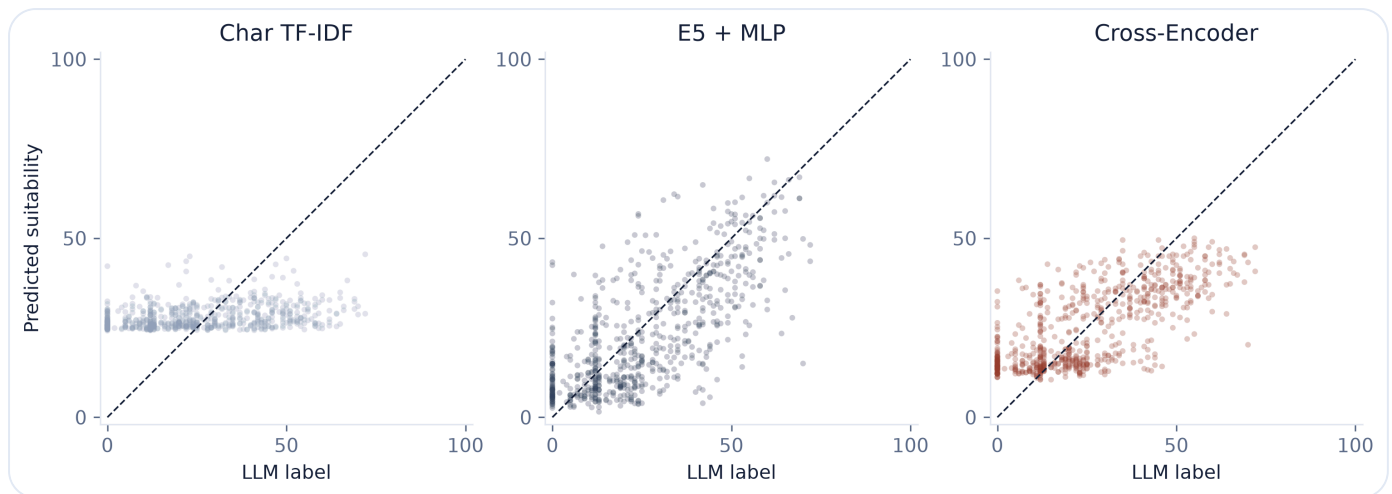
그림 9.3 LLM 라벨과 모델 예측값 (평가 분할 700쌍)
