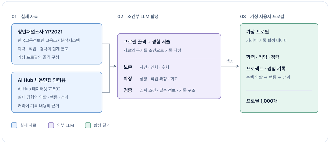
그림 3.2 실제 자료 기반 합성 프로필의 구축 과정
