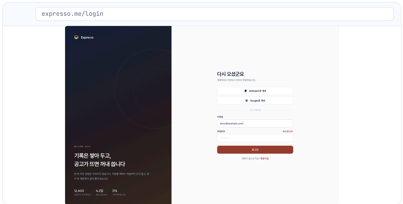
그림 5.3.25 로그인 (화면번호 10)
