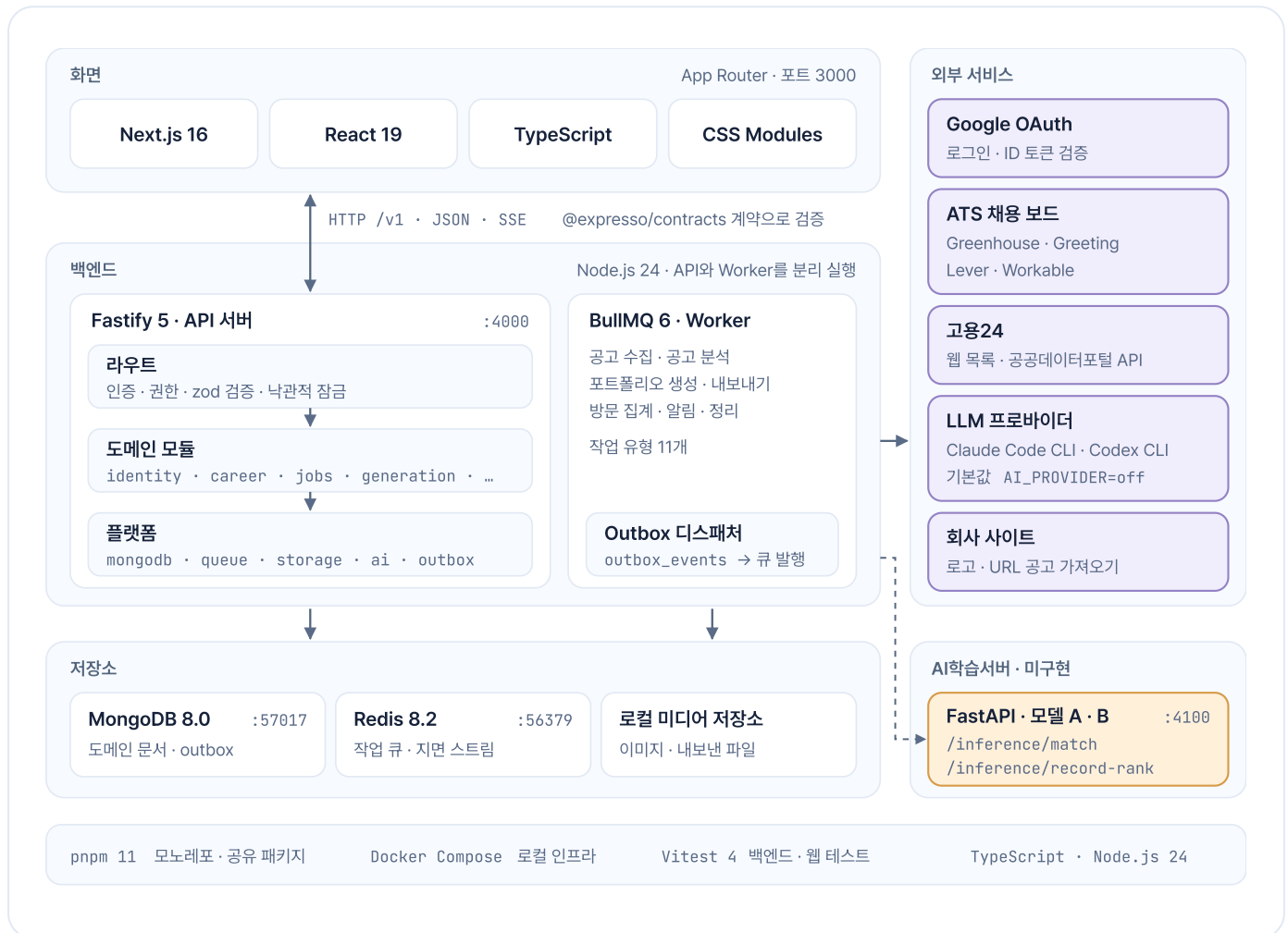
그림 6.1 시스템 아키텍처
