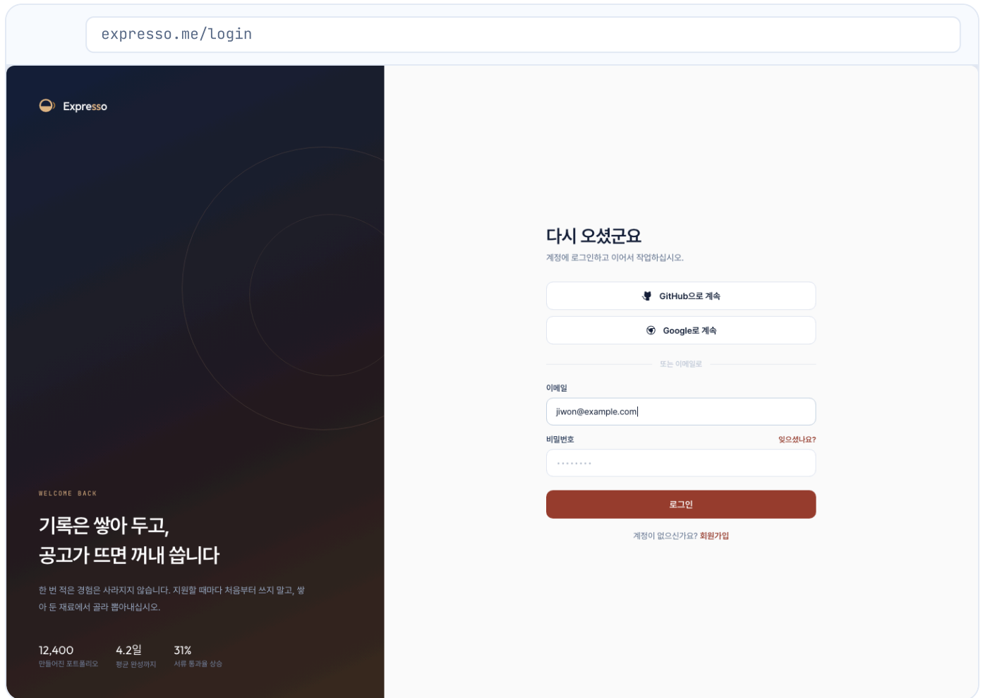
그림 5.2 초기화면(로그인) — 브라우저 프레임 포함 캡처
