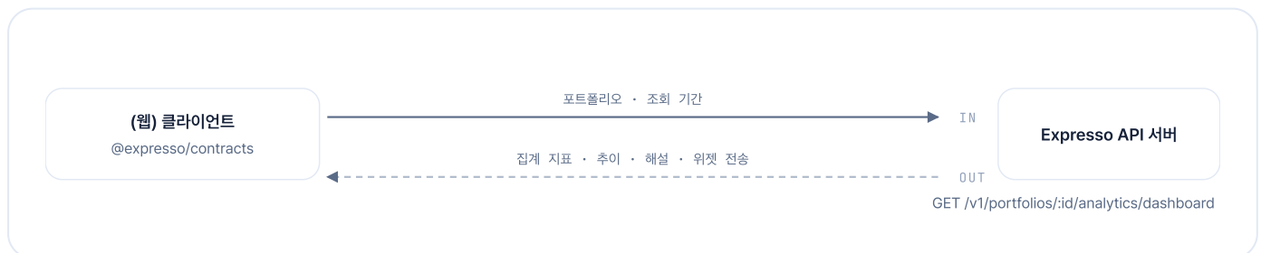
그림 7.3.24 분석 대시보드 조회의 요청·응답 방향
