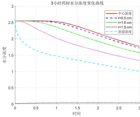
图 14 问题 2 3h 药材水分浓度变化曲线
