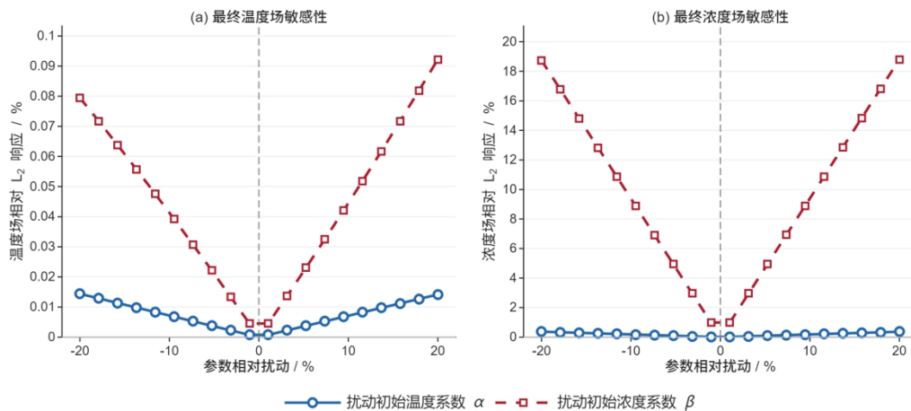
图 21 问题 2 初始条件敏感性分析
