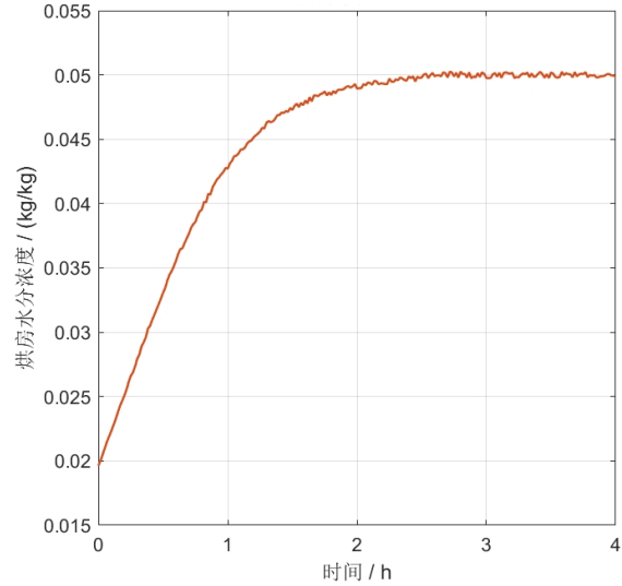
图4 烘房水分边界
