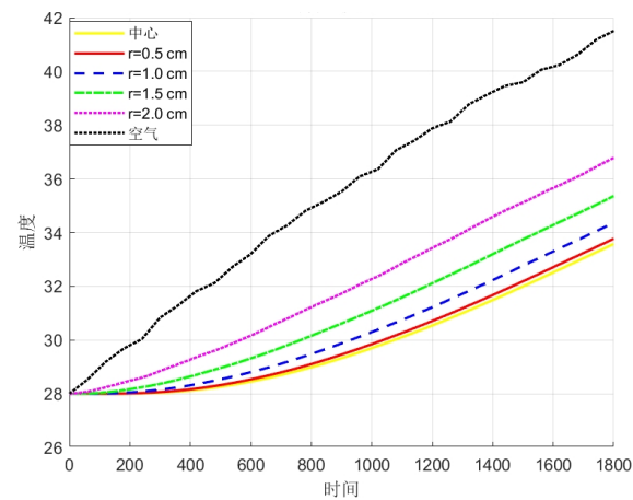
图 7 问题 1 药材温度变化图
