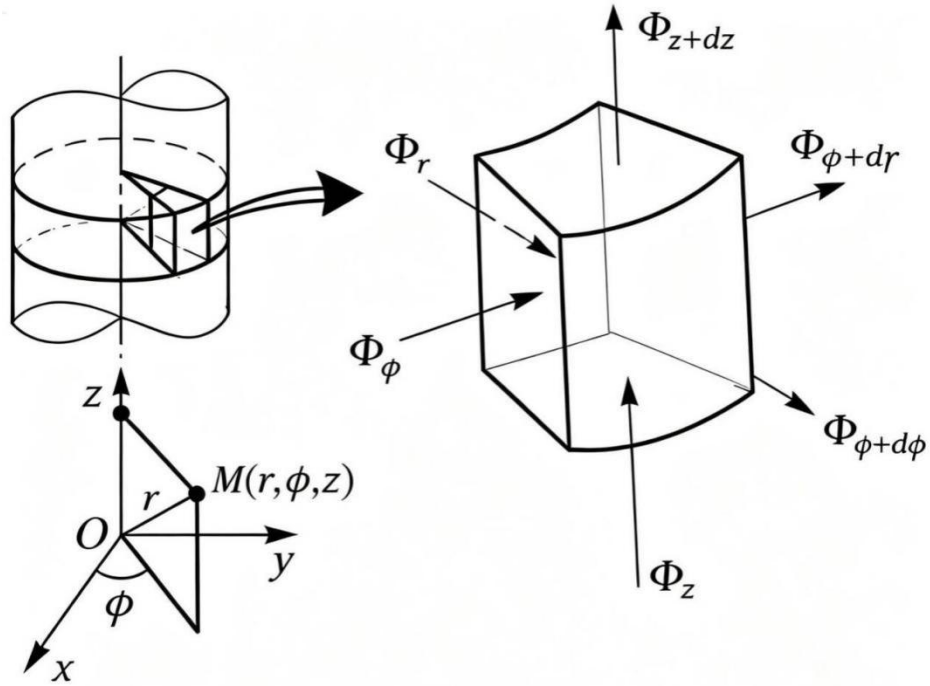
图 1 圆柱坐标系微元体
