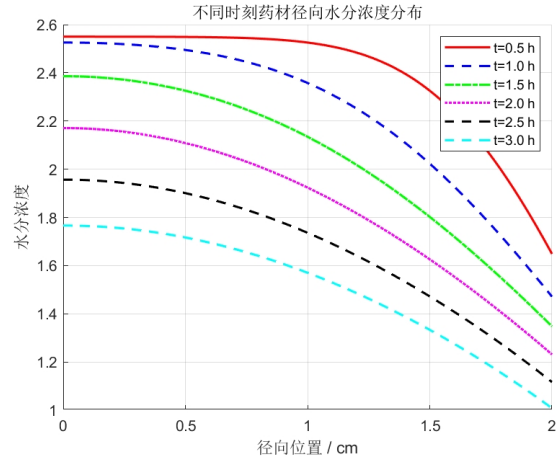
图 15 问题 2 不同时刻药材径向水分浓度分布
