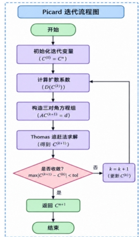
图 6 Picard 迭代流程图
