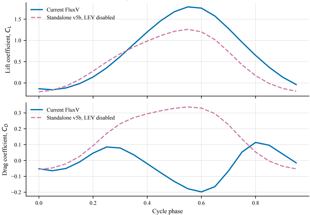
No-LEV reduction probe: Yang 2025, 15° nominal-four-bar smoke
