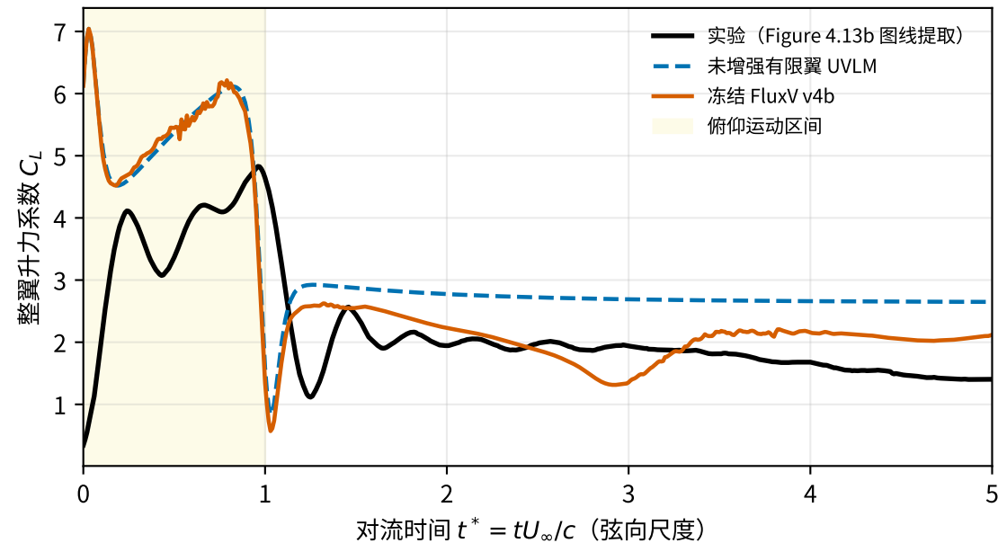
快速俯仰： s_a/c = 1 , k = 0.39
