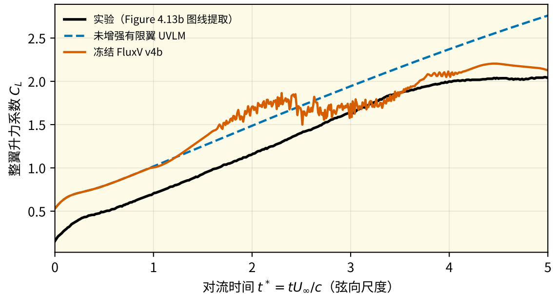
慢速俯仰： s_a/c = 6 , k = 0.065
