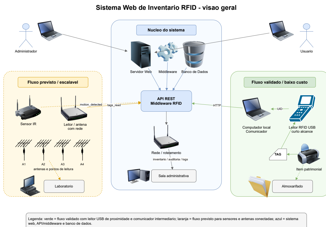
Figura 1 – Visão geral da arquitetura proposta para o sistema de inventário RFID
