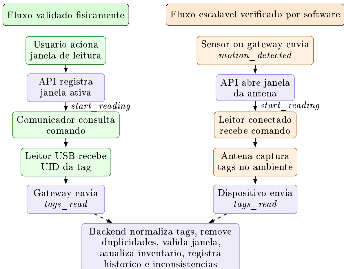
Figura 2 – Fluxo de eventos RFID suportado pela arquitetura
