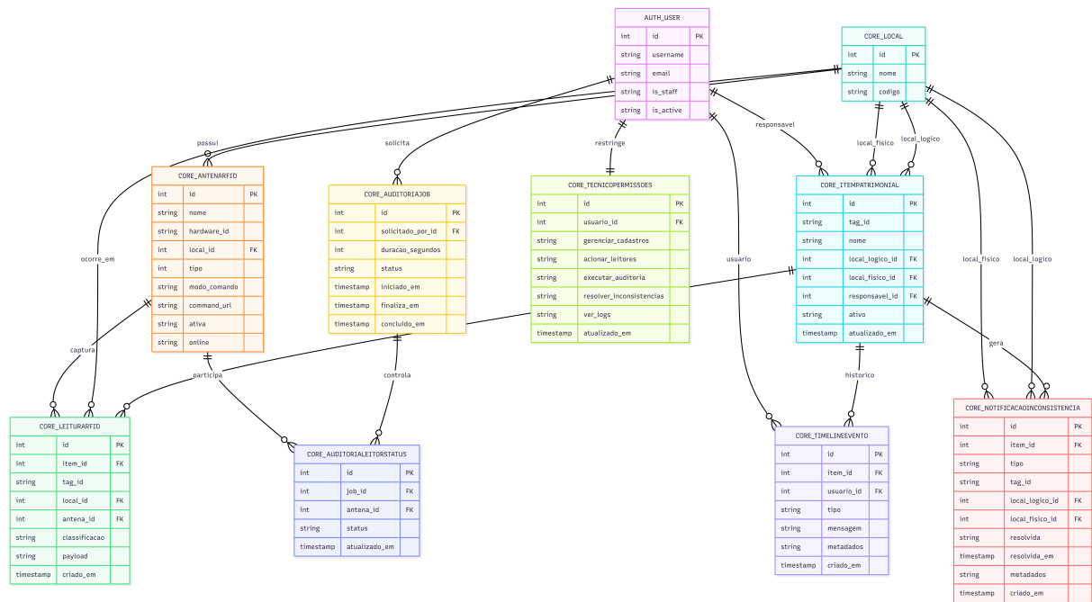
Figura 2 – Diagrama entidade-relacionamento do banco de dados do sistema de inventário RFID
