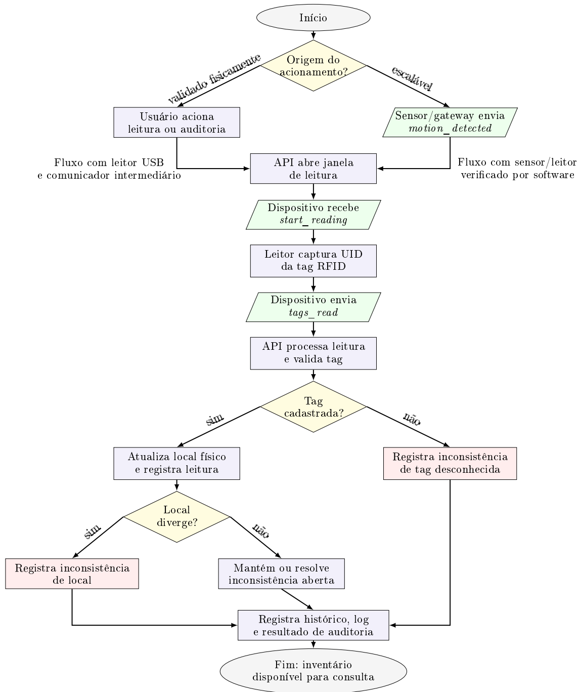
Figura 3 – Fluxograma geral para processamento de eventos RFID
