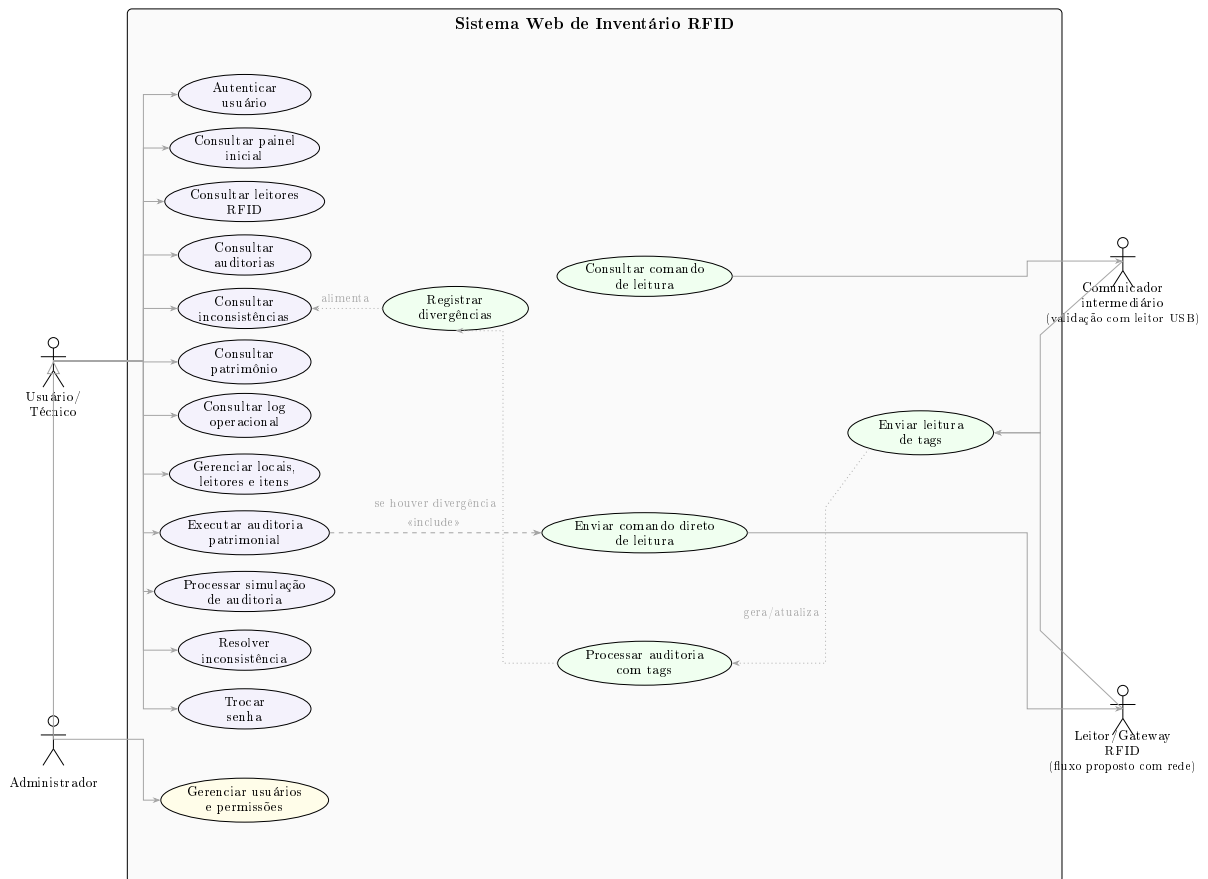
Figura 1 – Diagrama de casos de uso do sistema de inventário RFID
