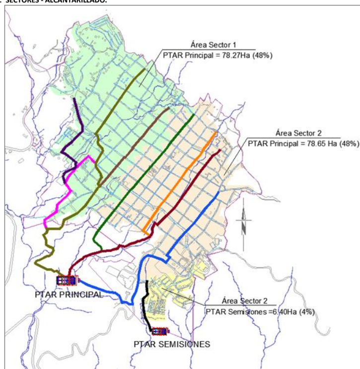
FIGURA 22: SECTORES - ALCANTARILLADO.
