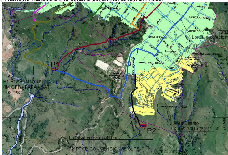
FIGURA 23: PLANTAS DE TRATAMIENTO DE AGUAS RESIDUALES DEFINIDAS EN EL PMAA.
