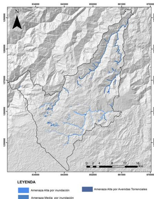
FIGURA 8: AMENAZAS POR INUNDACIÓN Y AVENIDAS TORRENCIALES EN EL TERRITORIO MUNICIPAL.
