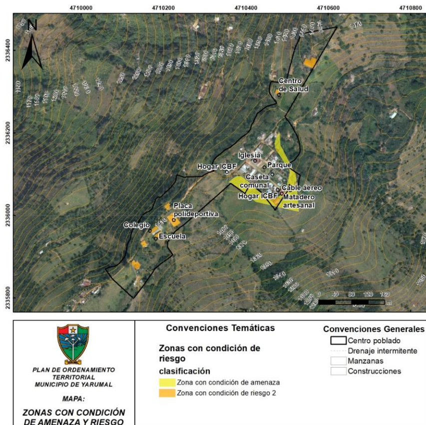
FIGURA 4. ÁREAS CON CONDICIÓN DE AMENAZA Y CON CONDICIÓN DE RIESGO EN EL CENTRO POBLADO RURAL DE LA LOMA.
