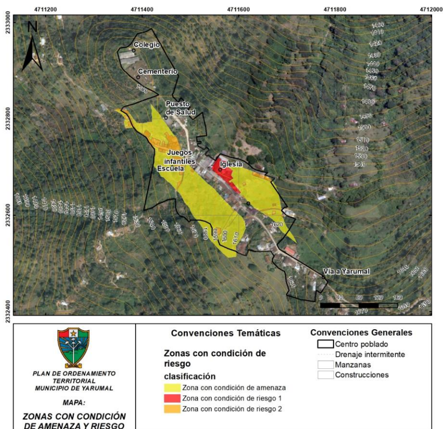
FIGURA 3. ÁREAS CON CONDICIÓN DE AMENAZA Y CON CONDICIÓN DE RIESGO EN EL CENTRO POBLADO RURAL DE OCHALÍ.
