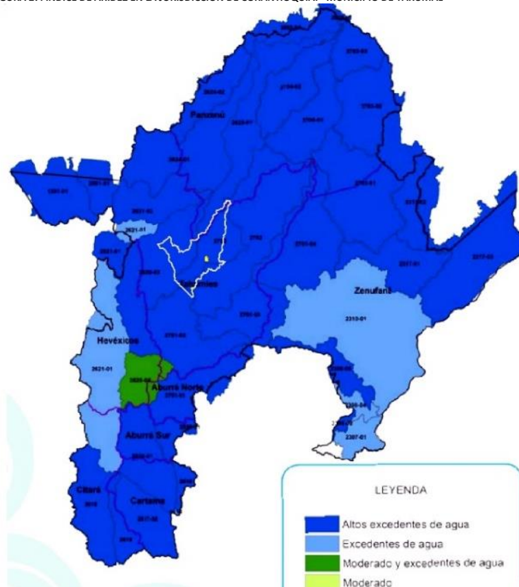
FIGURA 27. ÍNDICE DE ARIDÉZ EN LA JURISDICCIÓN DE CORANTIOQUIA. - MUNICIPIO DE YARUMAL
