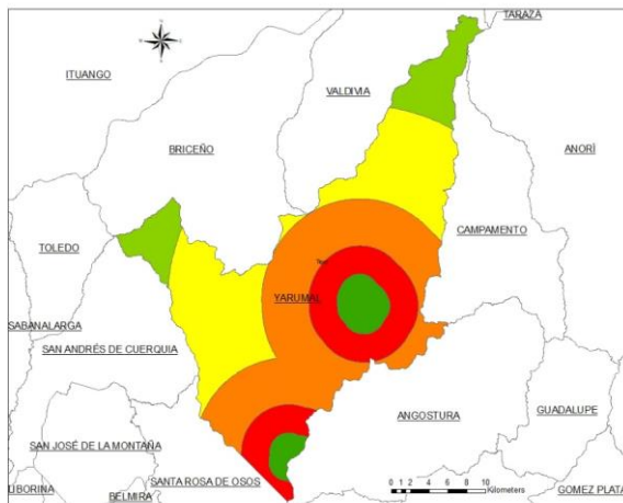
FIGURA 12. DISTANCIA A CENTROS POBLADOS
