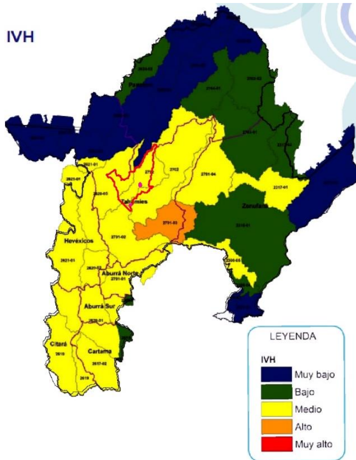
FIGURA 30. ÍNDICE DE VULNERABILIDAD HÍDRICA EN JURISDICCIÓN DE CORANTIOQUIA - MUNICIPIO DE YARUMAL.
