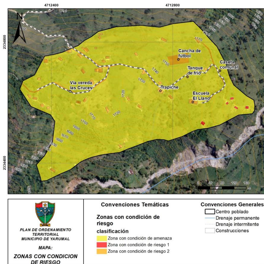
FIGURA 5. ÁREAS CON CONDICIÓN DE AMENAZA Y CON CONDICIÓN DE RIESGO EN EL CENTRO POBLADO RURAL DE EL LLANO.
