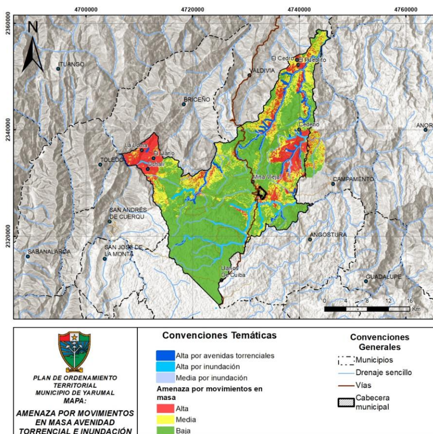
FIGURA 9. ÁREAS CON CONDICIÓN DE AMENAZA EN EL SUELO RURAL DEL MUNICIPIO DE YARUMAL.
