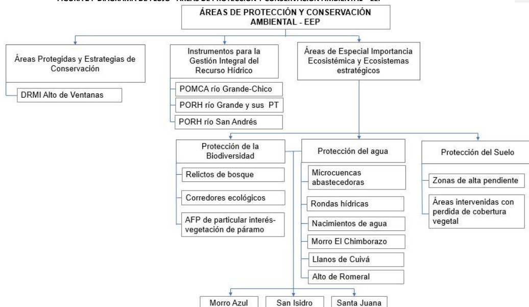
FIGURA 24 DIAGRAMA DE FLUJO - ÁREAS DE PROTECCIÓN Y CONSERVACIÓN AMBIENTAL - EEP
