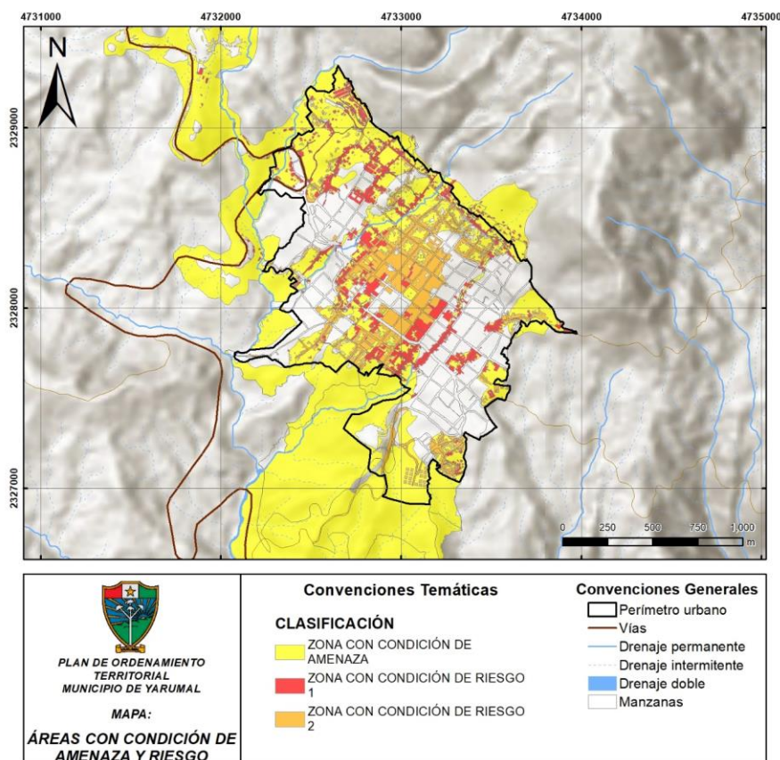
FIGURA 2. ÁREAS CON CONDICIÓN DE AMENAZA Y CON CONDICIÓN DE RIESGO EN LA CABECERA MUNICIPAL.
