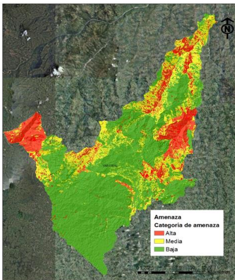
FIGURA 7: AMENAZAS NATURALES POR MOVIMIENTOS EN MASA EN EL TERRITORIO MUNICIPAL.
