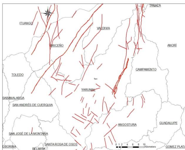
FIGURA 15. DISTANCIA A FALLAS GEOLÓGICAS
