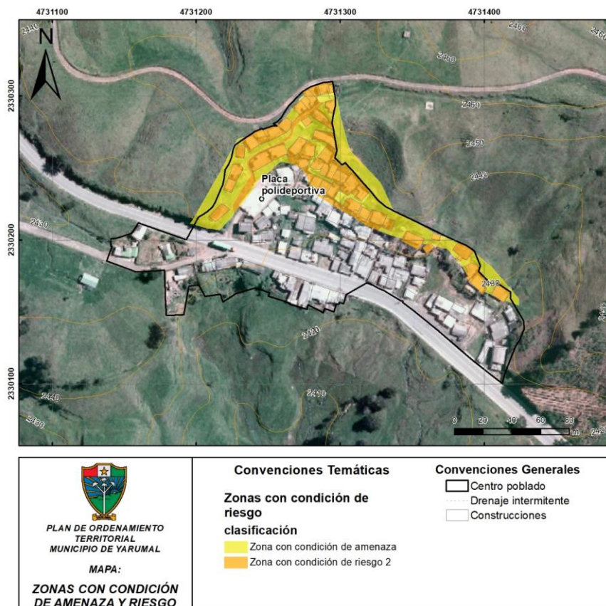
FIGURA 6. ÁREAS CON CONDICIÓN DE AMENAZA Y CON CONDICIÓN DE RIESGO EN EL CENTRO POBLADO RURAL DE MINA VIEJA.
